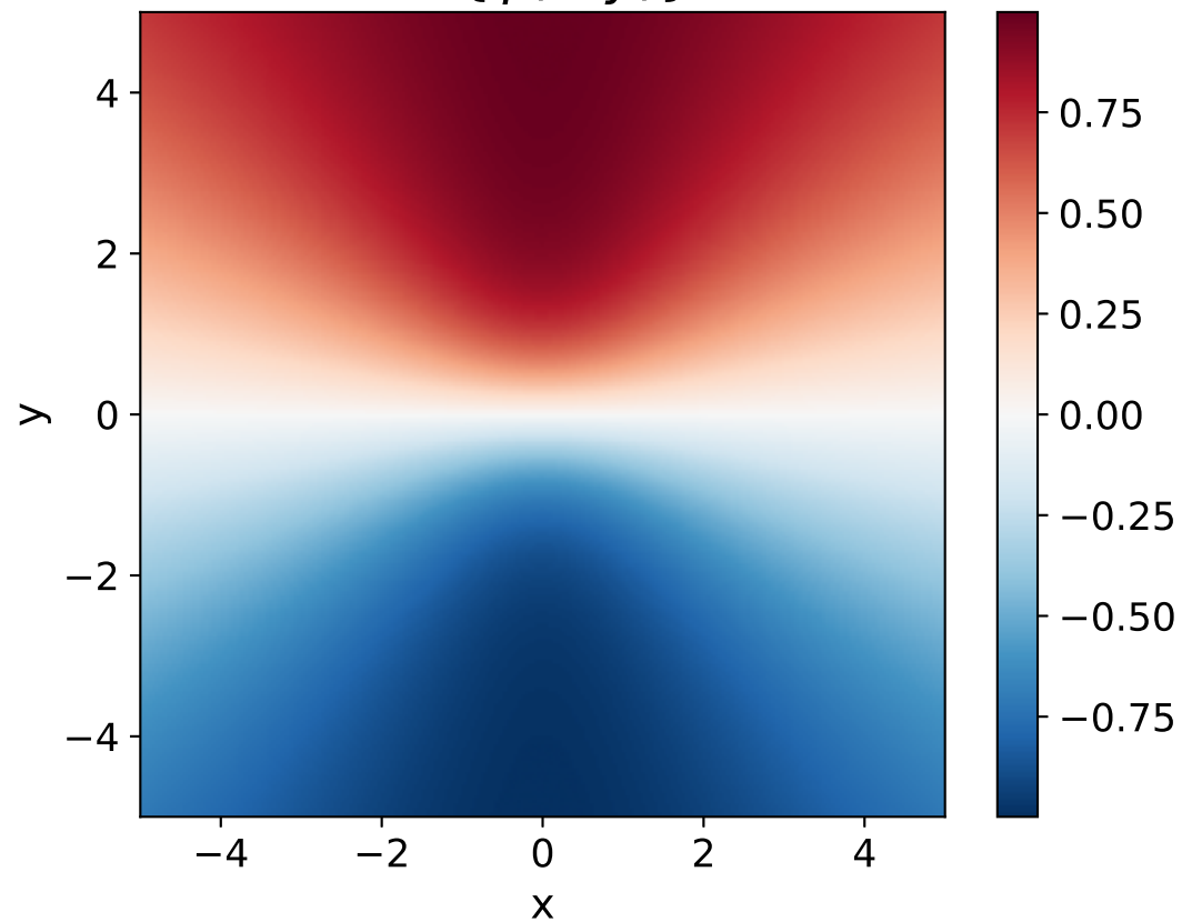
\arg\{\psi(x, y)/\pi\}
