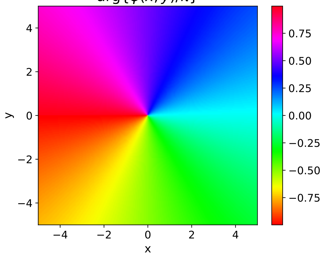
\arg\{\psi(x, y)/\pi\}
