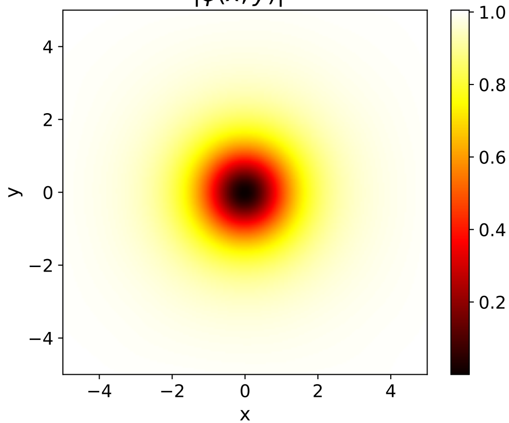
|\psi(x, y)|^2
