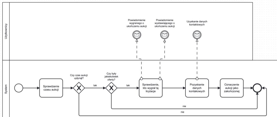
Rysunek 5.3: Kończenie aukcji
