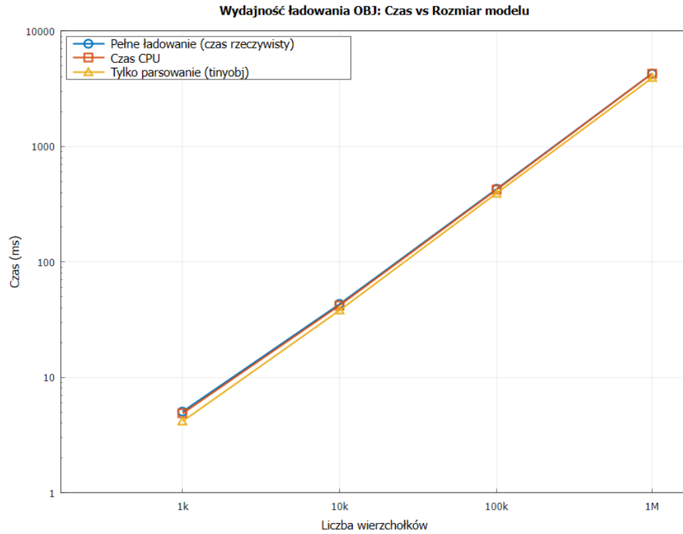
Rysunek 12.2: Zależność czasu ładowania od rozmiaru modelu (skala logarymiczna)
