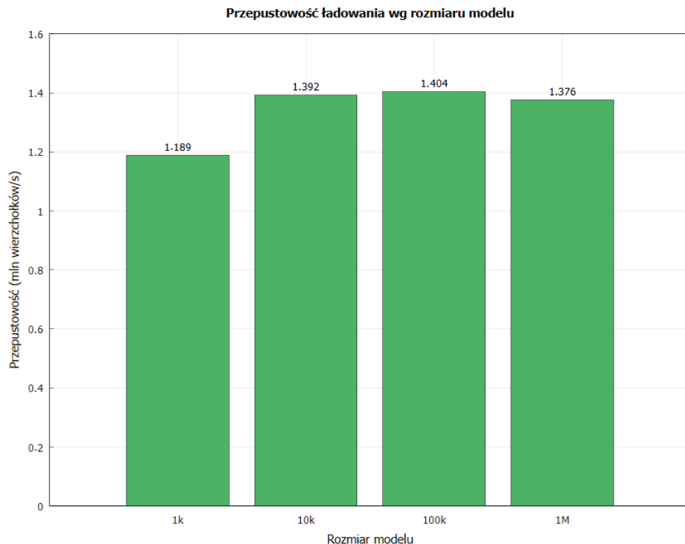
Rysunek 11.4: Przepustowość ładowania modeli OBJ
