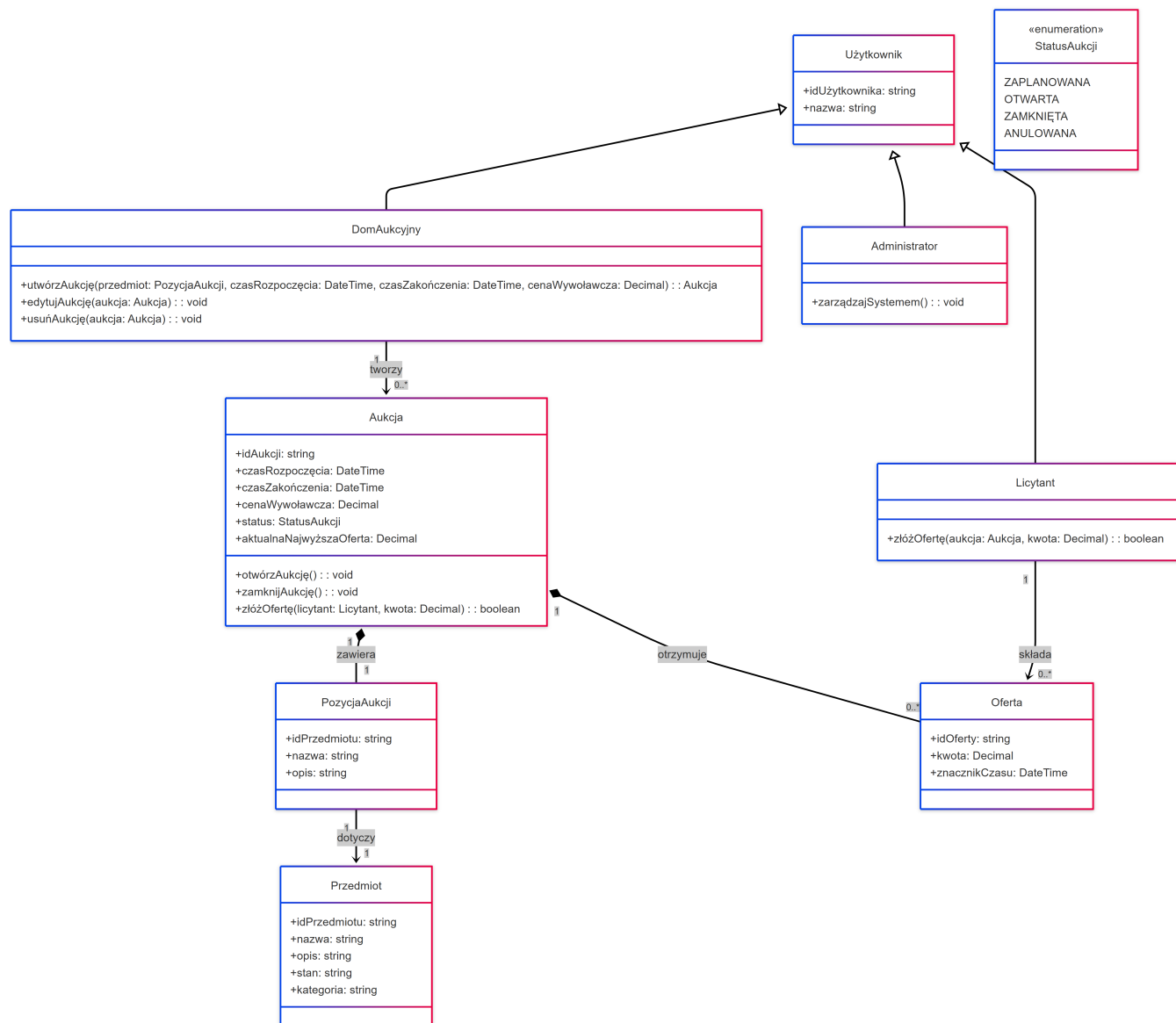
Rysunek 5.10: Diagram klas procesu licytacji
