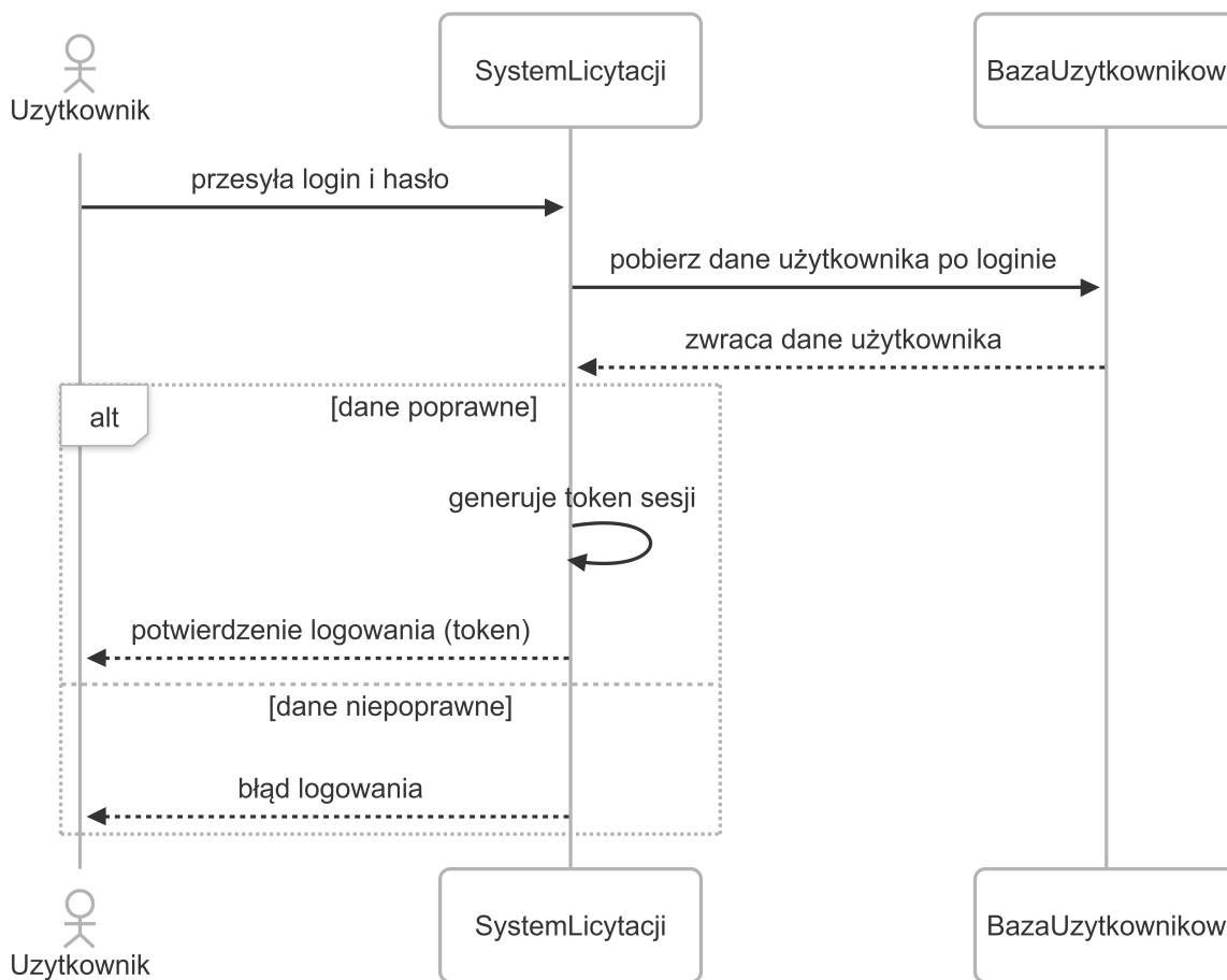
Rysunek 5.13: Logowanie
