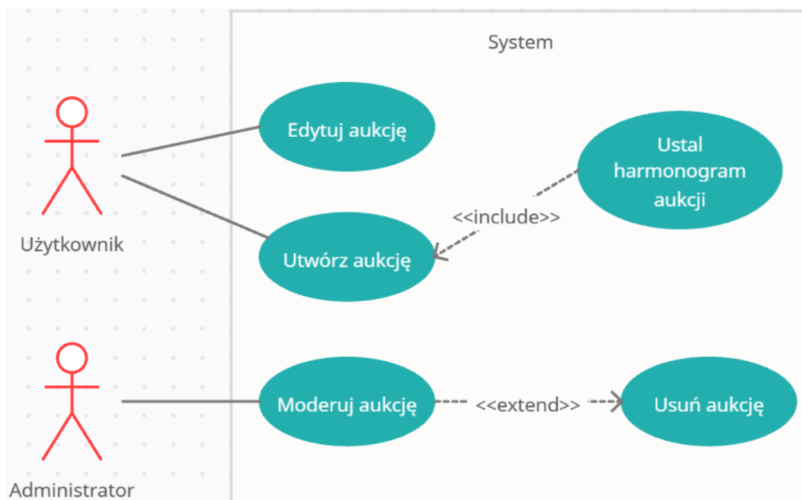
Rysunek 6.6: Diagram przypadków użycia zarządzania aukcjami
