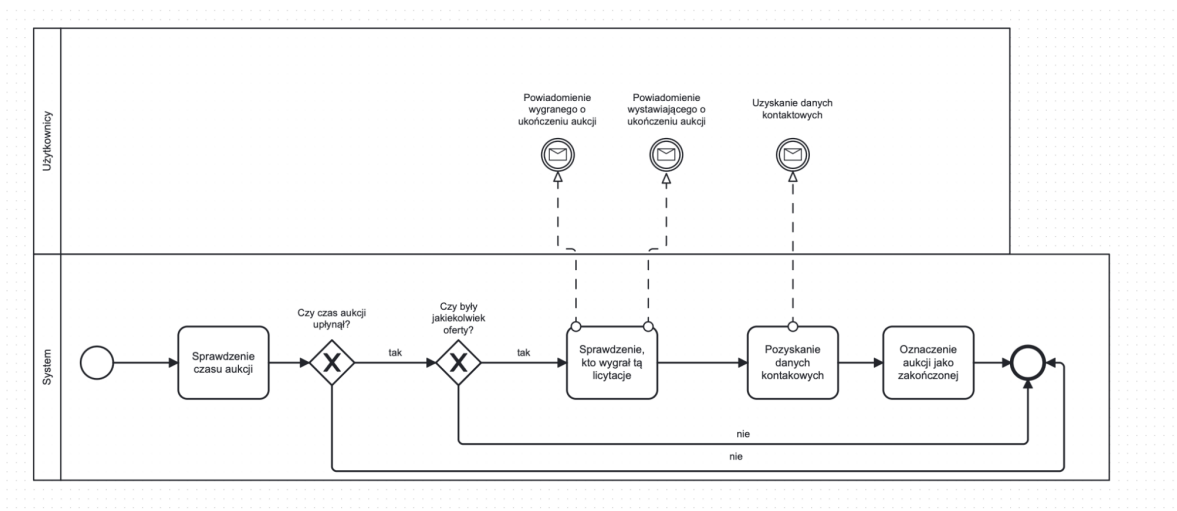
Rysunek 6.3: Diagram BPMN - kończenie aukcji
