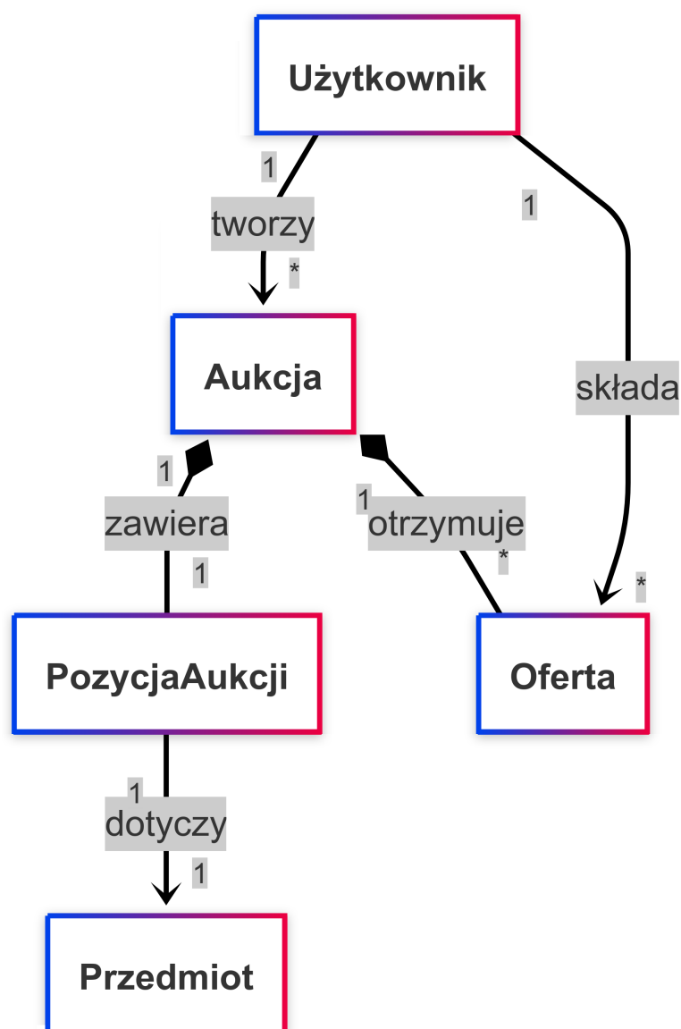
Rysunek 6.20: Model danych - uproszczony diagram klas
