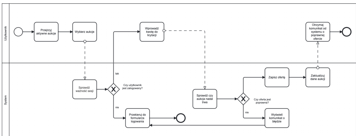
Rysunek 6.2: Diagram BPMN - proces licytacji
