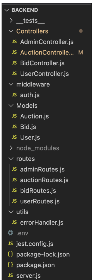
Rysunek 10.1: Struktura części serwerowej systemu aukcyjnego
