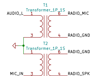
Transformateurs
