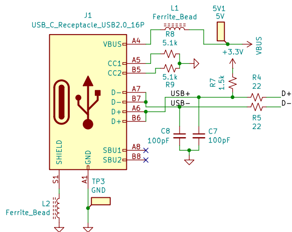
Connecteur USB
