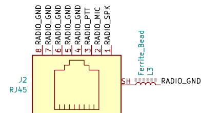
Connecteur RJ45
