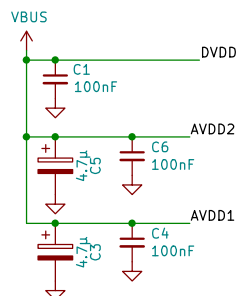
Condensateurs de découplage
