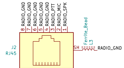
Connecteur RJ45
