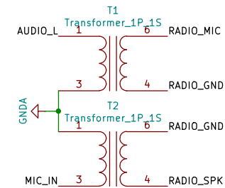
Transformateurs
