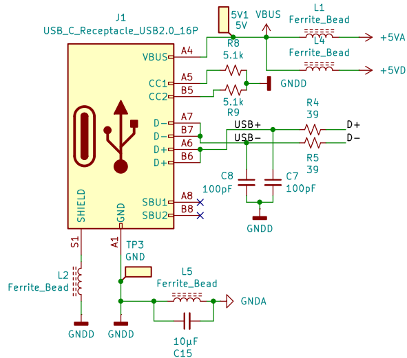
Connecteur USB
