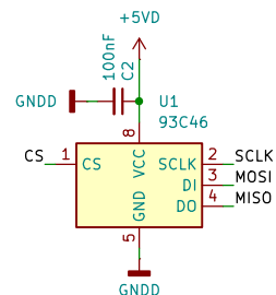
EEPROM
