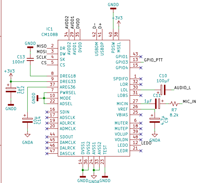
IC Audio
