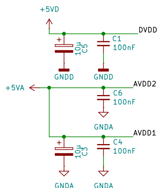
Condensateurs de découplage
