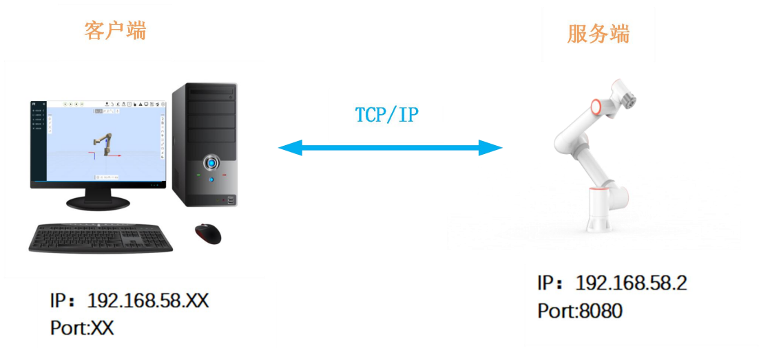
图 1-1 系统框图
