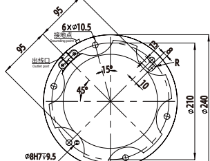
FR30 基座图 Pedestal diagram
