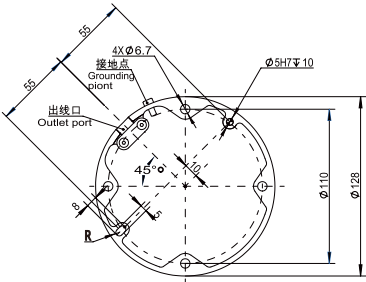
FR3-WMS 基座图 Pedestal diagram
