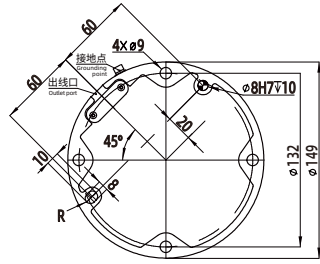
FR5 基座图 Pedestal diagram
