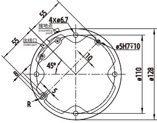
FR3 基座图 Pedestal diagram
