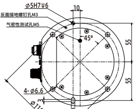
FR3-C 基座图 Pedestal diagram
