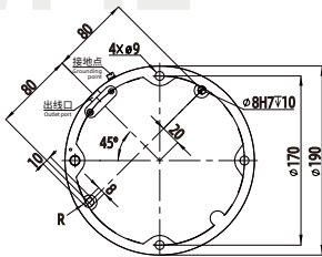
FR5-WML 基座图 Pedestal diagram
