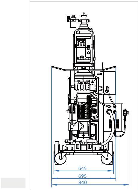
技术图纸 单位: mm
