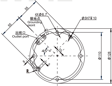
FR3-WML 基座图 Pedestal diagram
