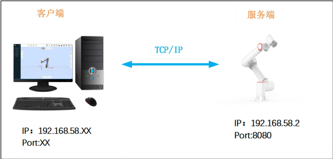
图 1-1 系统框图
