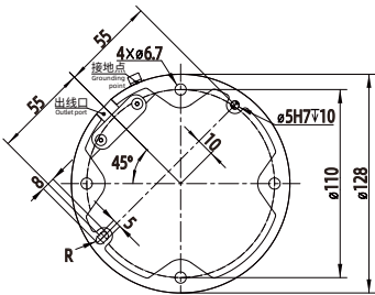
FR3 基座图 Pedestal diagram
