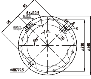
FR30 基座图 Pedestal diagram
