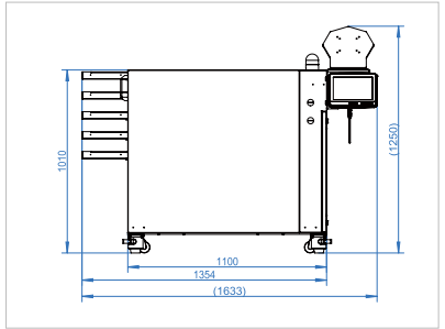
技术图纸 单位: mm
