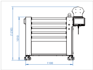
技术图纸 单位: mm
