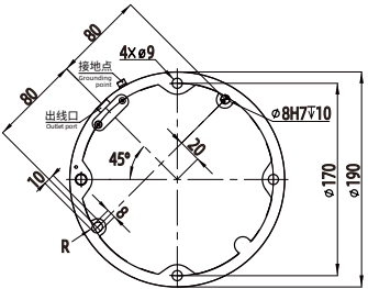
FR10 基座图 Pedestal diagram
