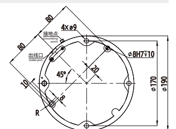
FR5-WML 基座图 Pedestal diagram
