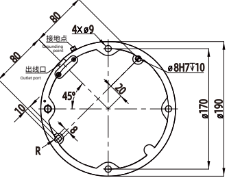
FR16 基座图 Pedestal diagram
