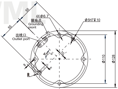
FR3-WML 基座图 Pedestal diagram
