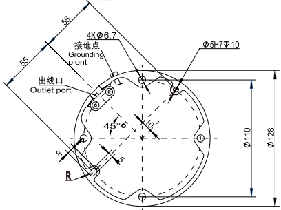
FR3-WMS 基座图 Pedestal diagram
