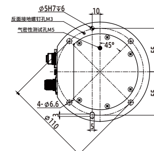
FR5-C 基座图 Pedestal diagram
