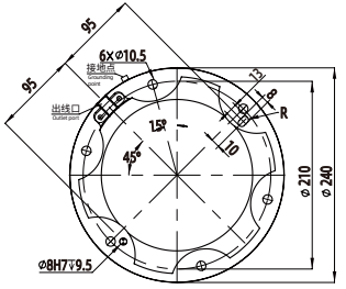
FR20 基座图 Pedestal diagram
