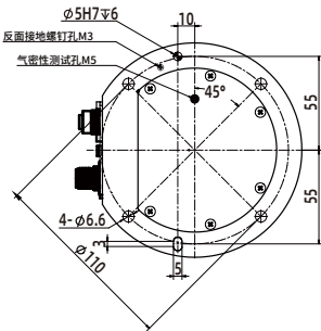
FR3-C 基座图 Pedestal diagram
