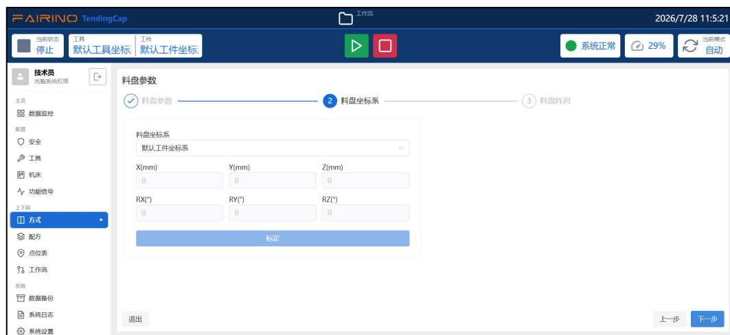
图 8.1-3 料盘坐标系
