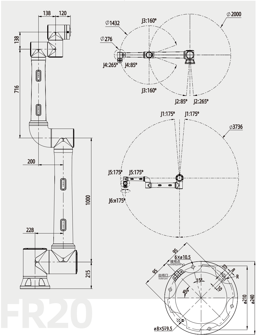
FR20 基座图 Pedestal diagram
