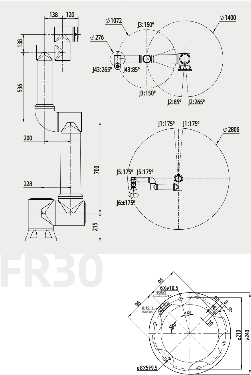
FR30 基座图 Pedestal diagram
