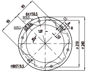
FR20 基座图 Pedestal diagram
