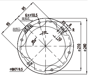
FR30 基座图 Pedestal diagram
