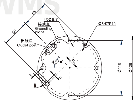
FR3WMS 基座图
