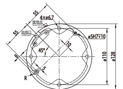
FR3 基座图 Pedestal diagram
