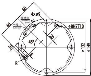
FR5 基座图 Pedestal diagram
