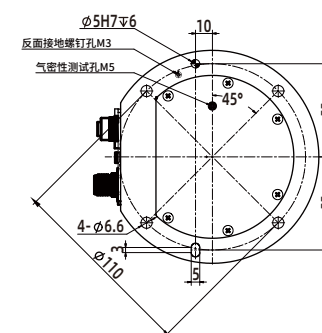
FR3C 基座图 Pedestal diagram
