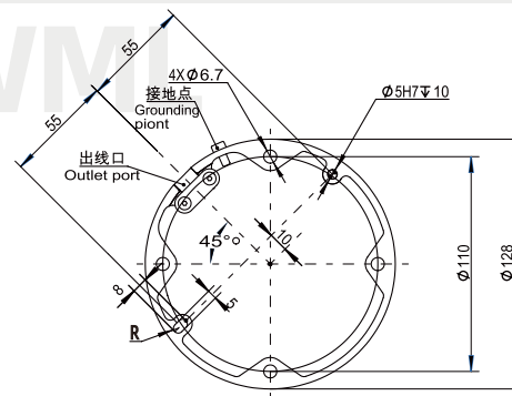
FR3WML 基座图 Pedestal diagram
