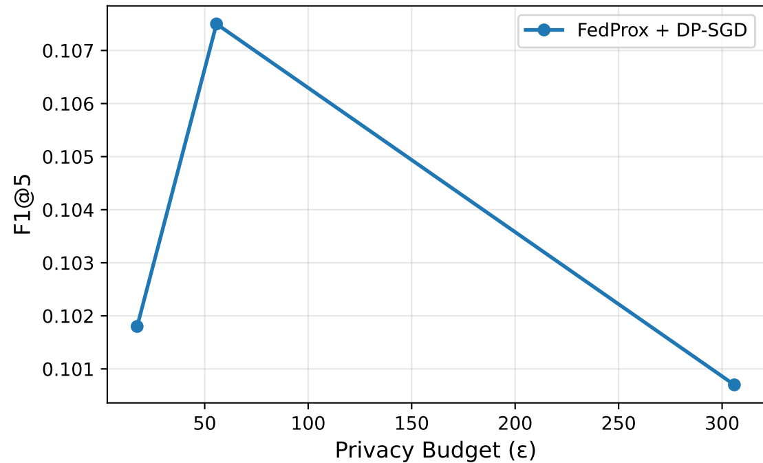
Privacy-Utility Tradeoff (FedProx + DP-SGD)
