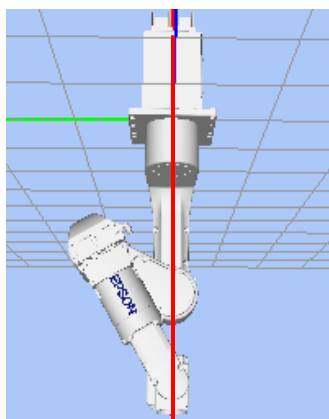
Singularidad de mano
