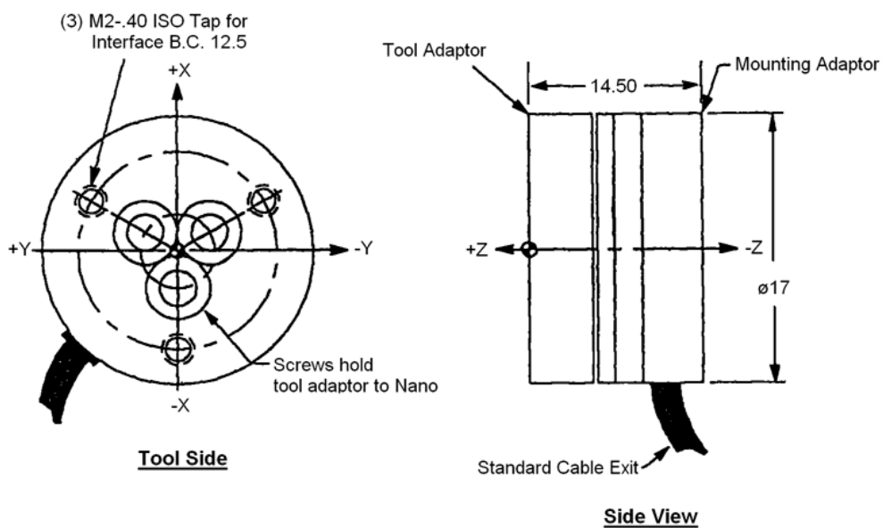
Montaje de herramientas para el transductor Nano
