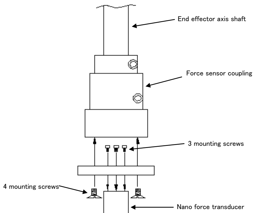
Montaje del sensor de fuerza Nano
