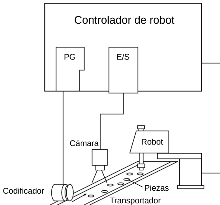
Descripción general del seguimiento del transportador con visión (uso de un desencadenador de software)
