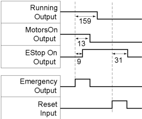
Diagrama de temporización para la secuencia de la parada de emergencia
