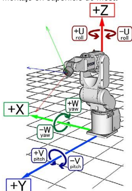
Montaje en superficie de mesa
