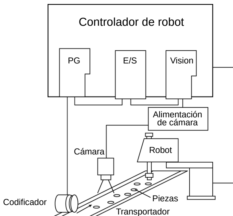
Descripción general del seguimiento del transportador con visión (uso de un desencadenador de hardware)
