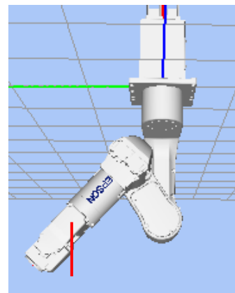
Singularidad de muñeca
