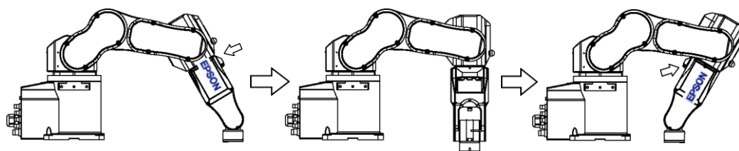
Movimiento no intencional (las uniones n.º 4 y 6 giran en 180 grados)
