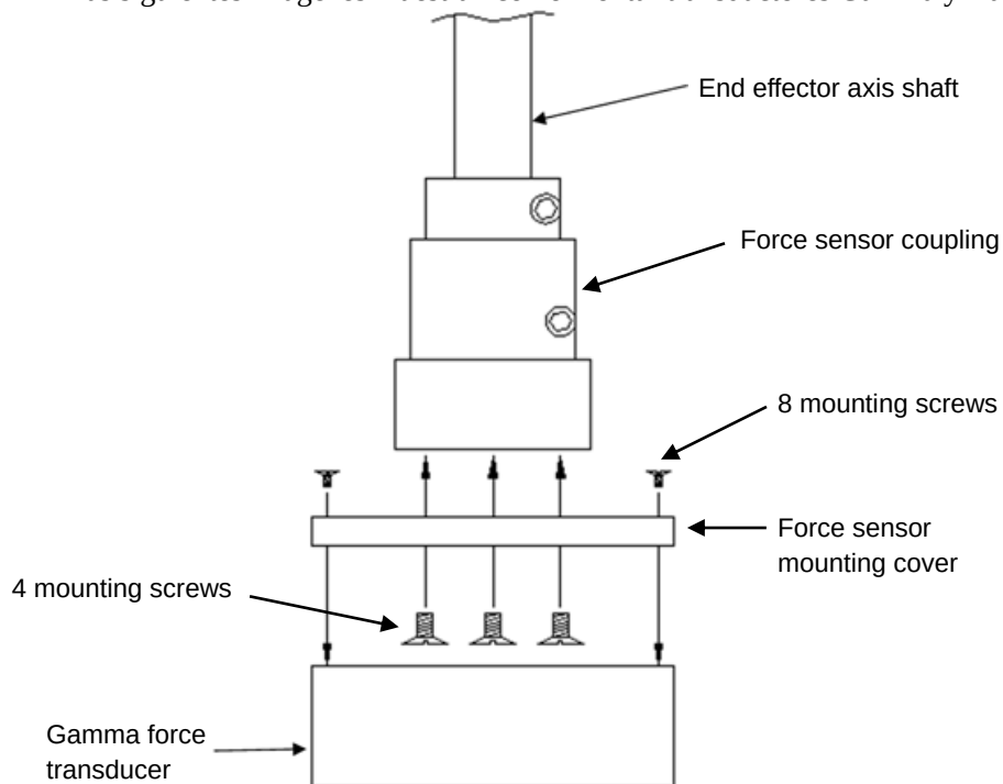
Montaje del sensor de fuerza Gamma
