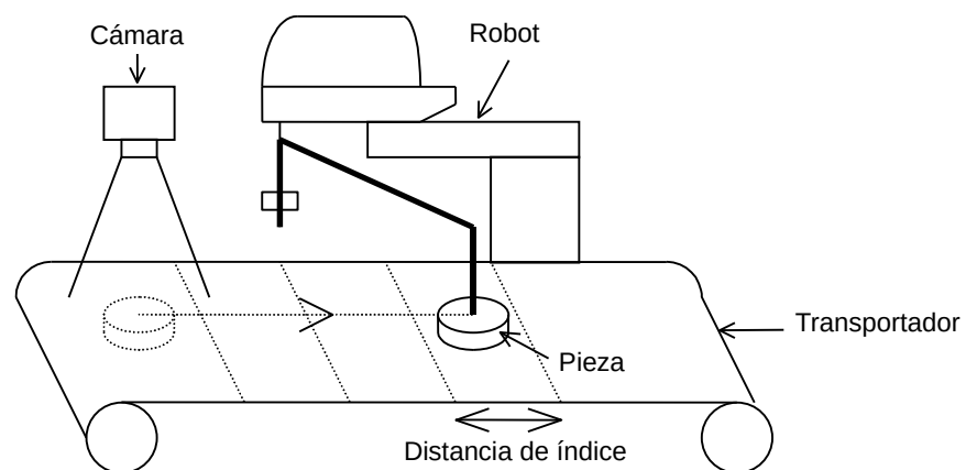
Sistema de transportador indizado
