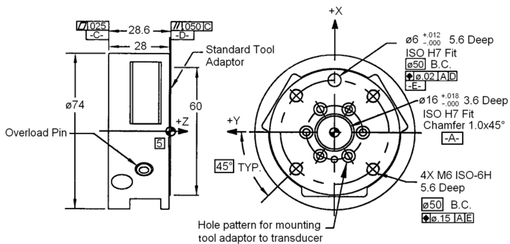
Montaje de herramientas para el transductor Gamma
