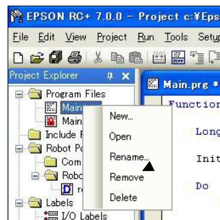
Menú contextual
