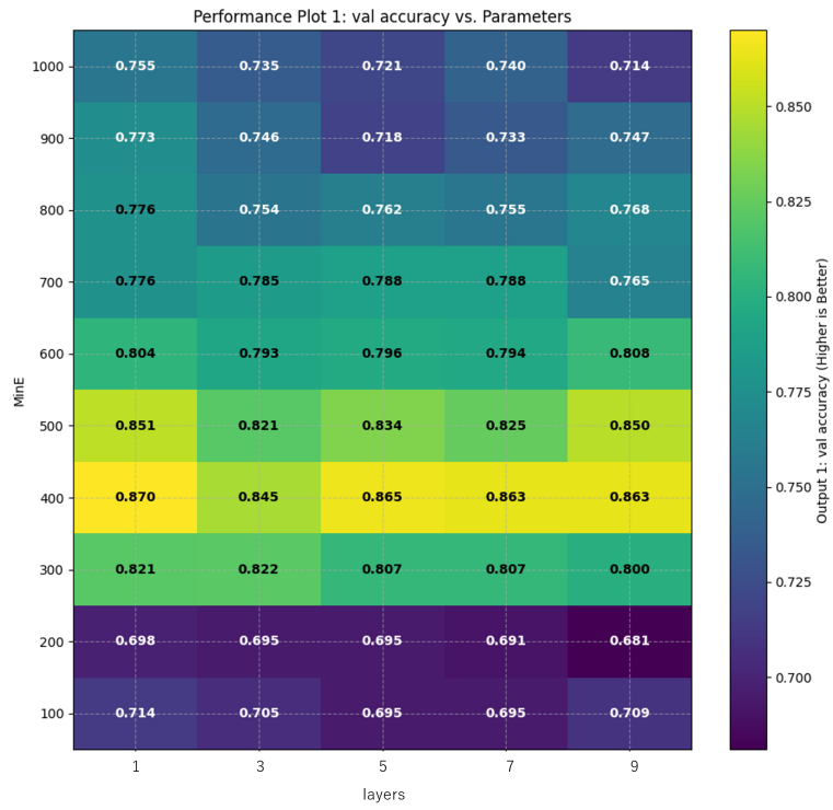
図 7.2 タスク 1 の学習結果 ( E_c=20 TeV)
