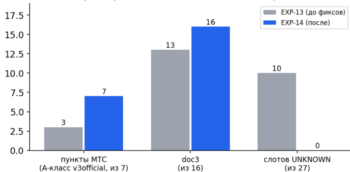
Три дыры, найденные бенчем, и их закрытие
