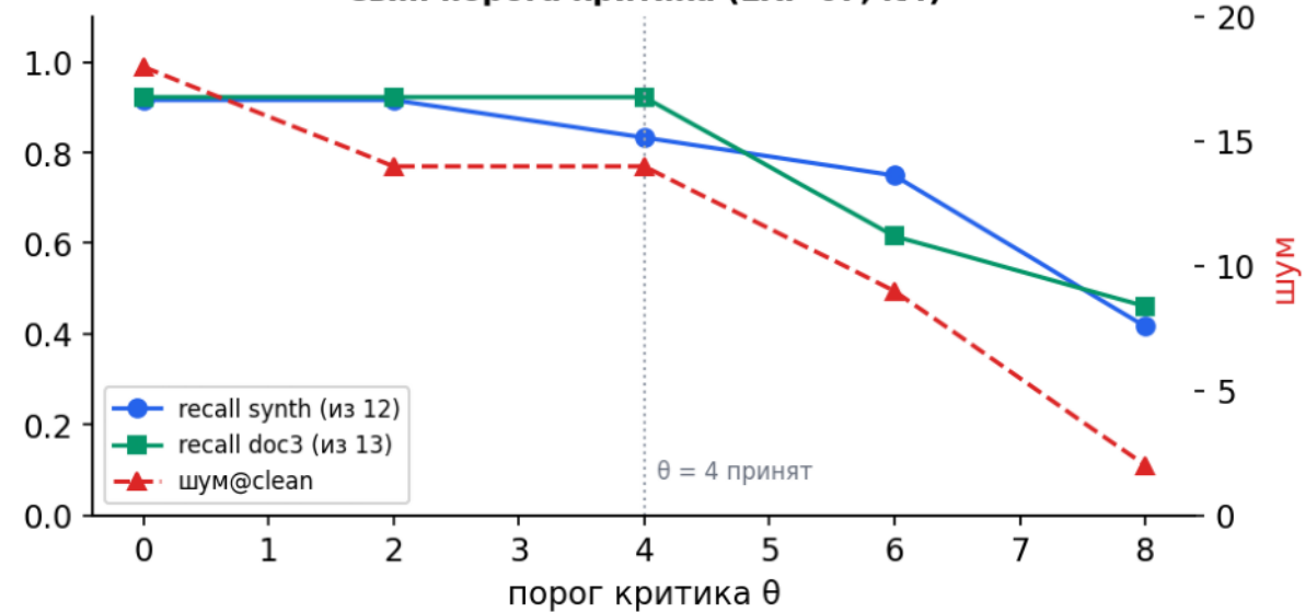
Свип порога критика (EXP-07, it4)
