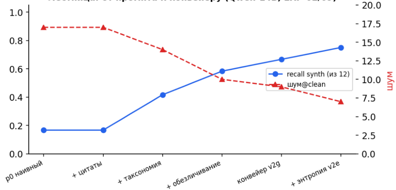
Лестница: от промпта к конвейеру (Qwen-14B, EXP-02/09)
