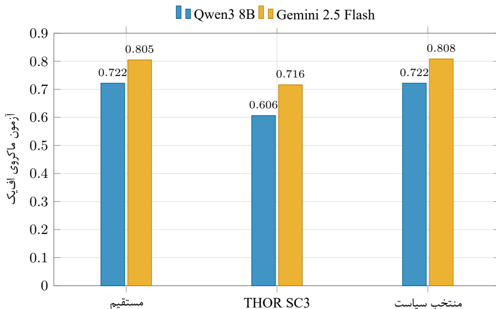
شکل ۵-۳: مقایسه امتیاز افیک ماکرو Qwen3 8B و Gemini 2.5 Flash روی زیرمجموعه مشترک ۹۰ نمونه‌ای آزمون.
