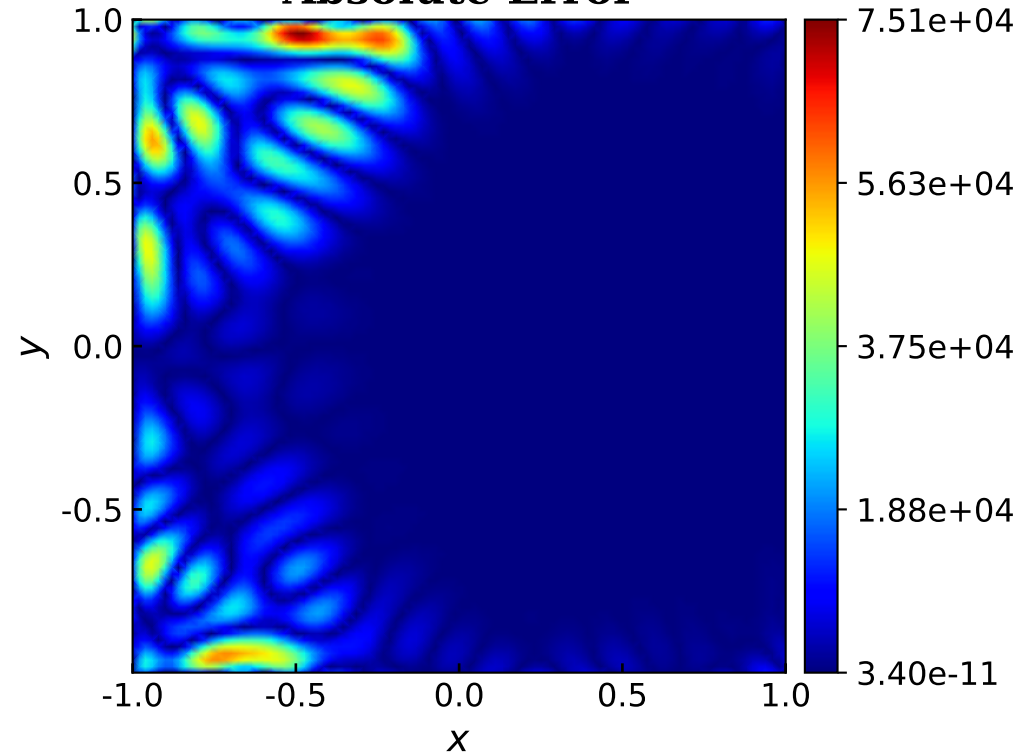
Absolute Error
