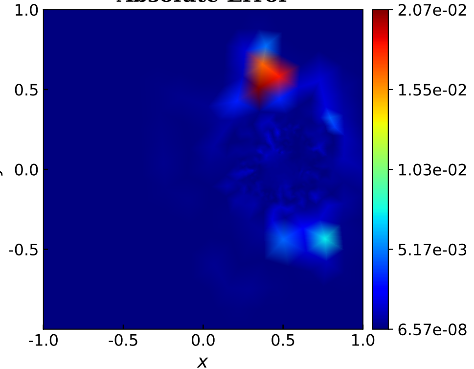
Absolute Error
