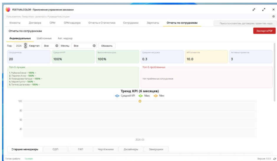
Отчёты по сотрудникам — KPI-дашборд и рейтинги
