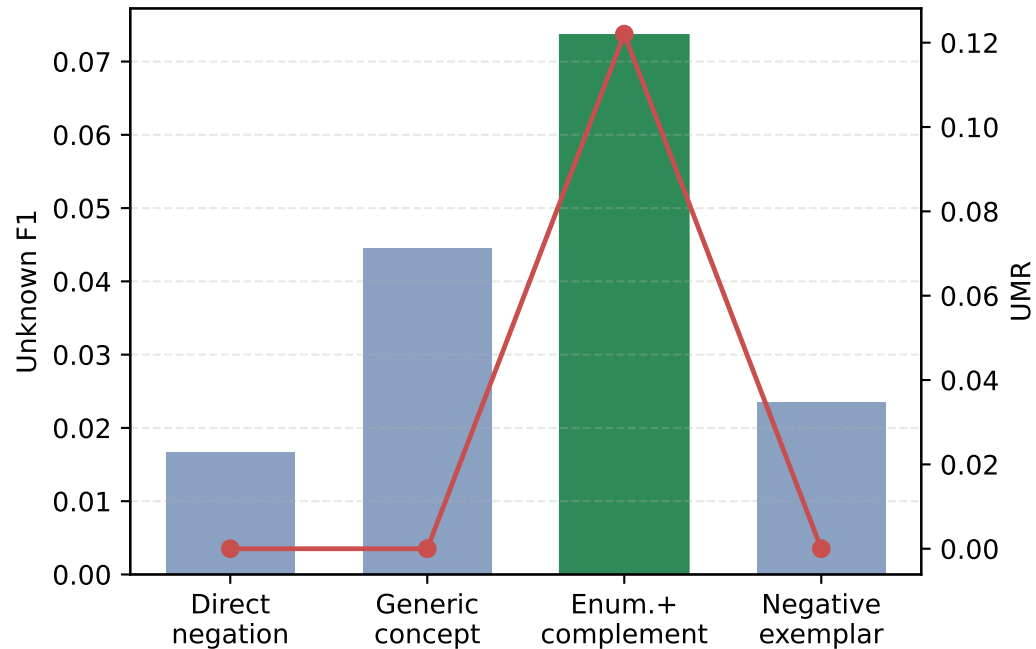
Cityscapes
