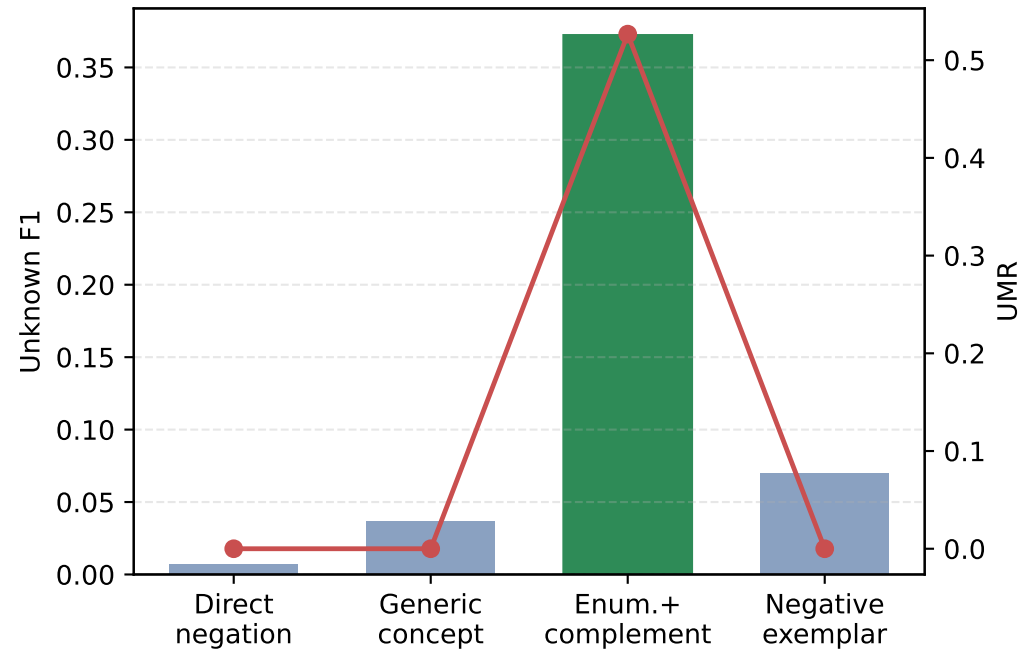
VOC
