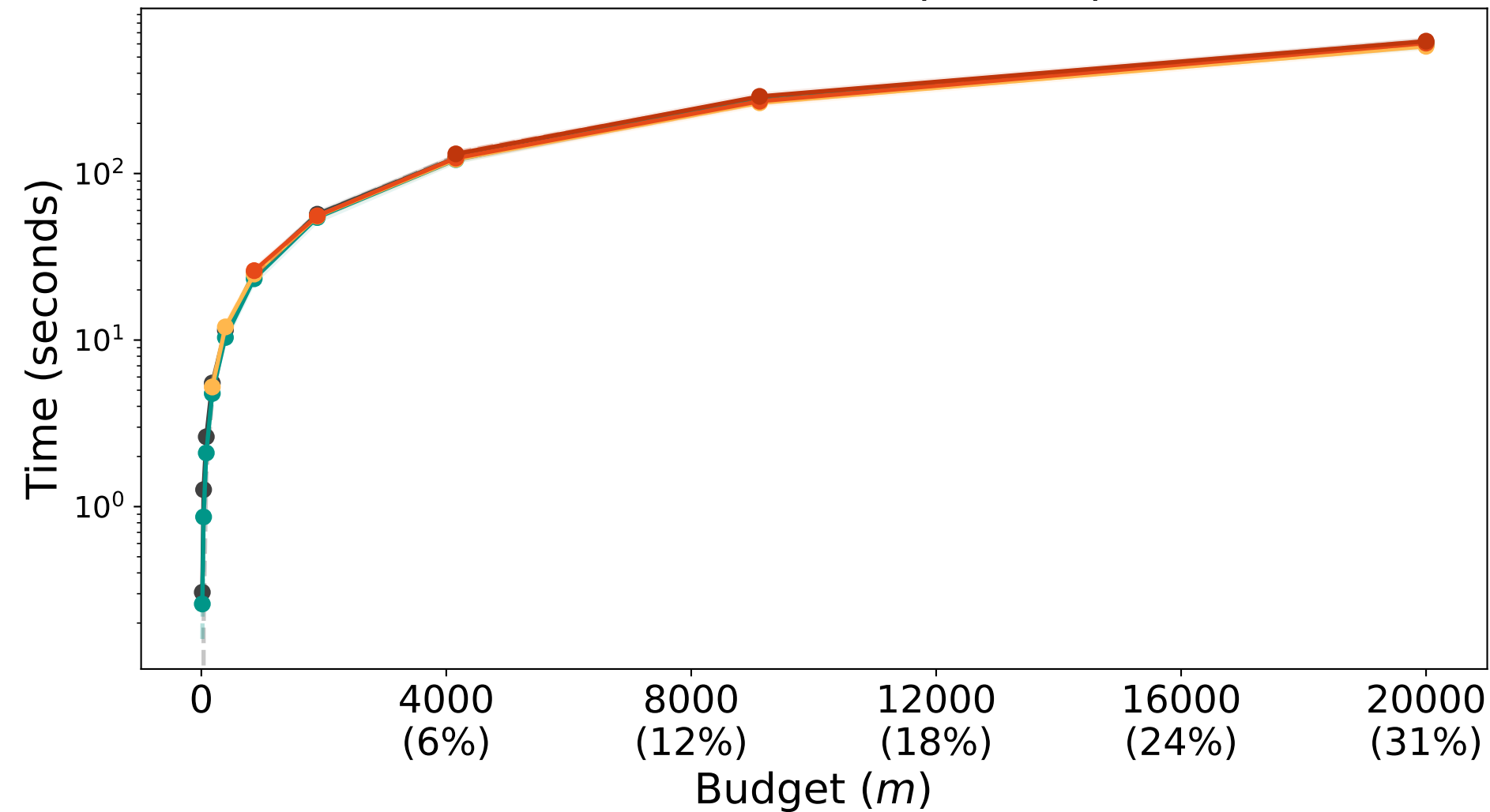
CIFAR10-ViT16 ( d = 16 )
