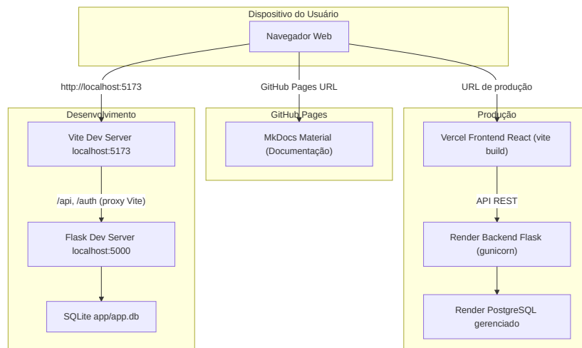
Figura 8: Diagrama de implantação.
