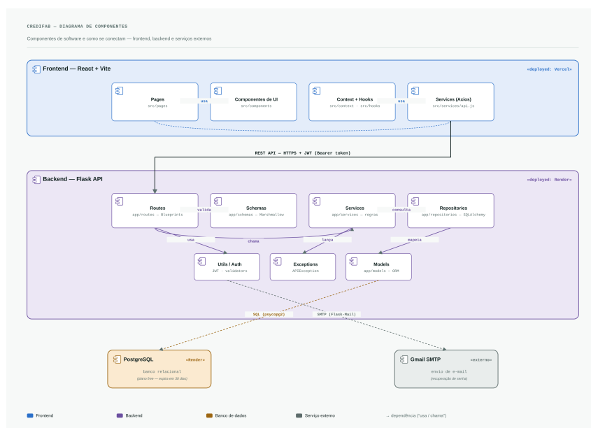
Figura 6: Diagrama dos componentes.
