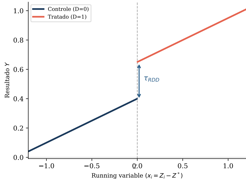
(A) Sharp RDD: salto no nível
