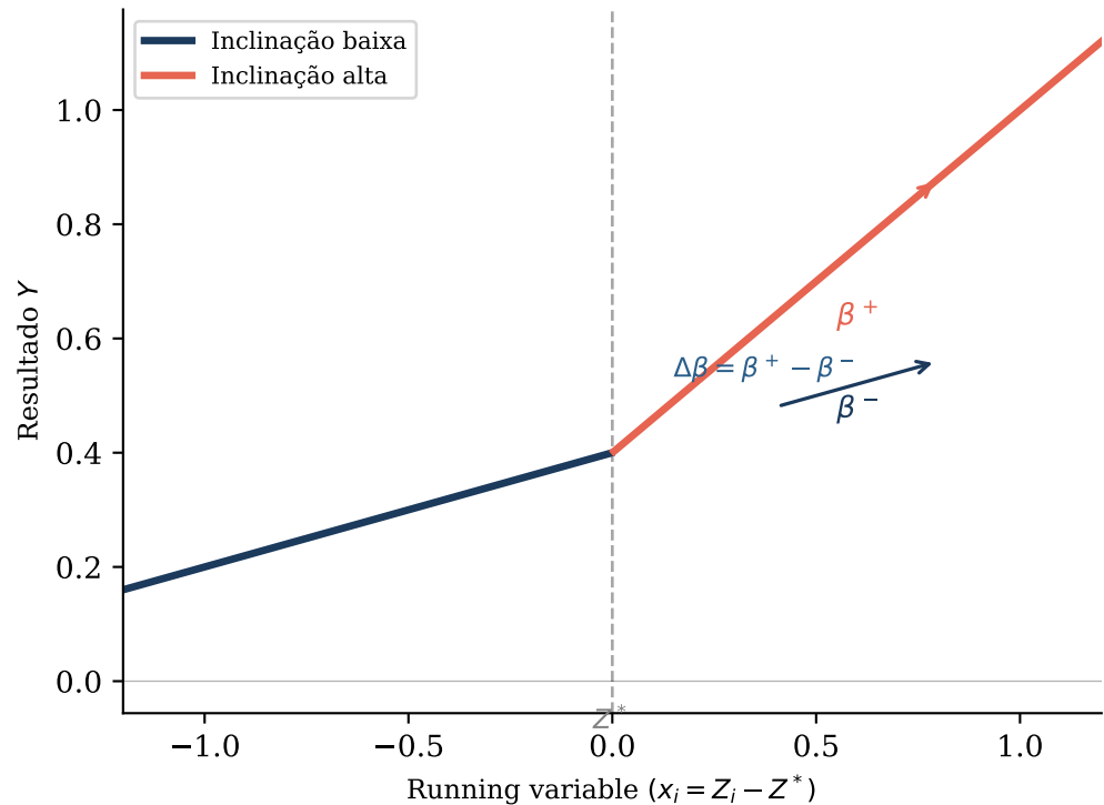
(B) RKD: quina na inclinação
