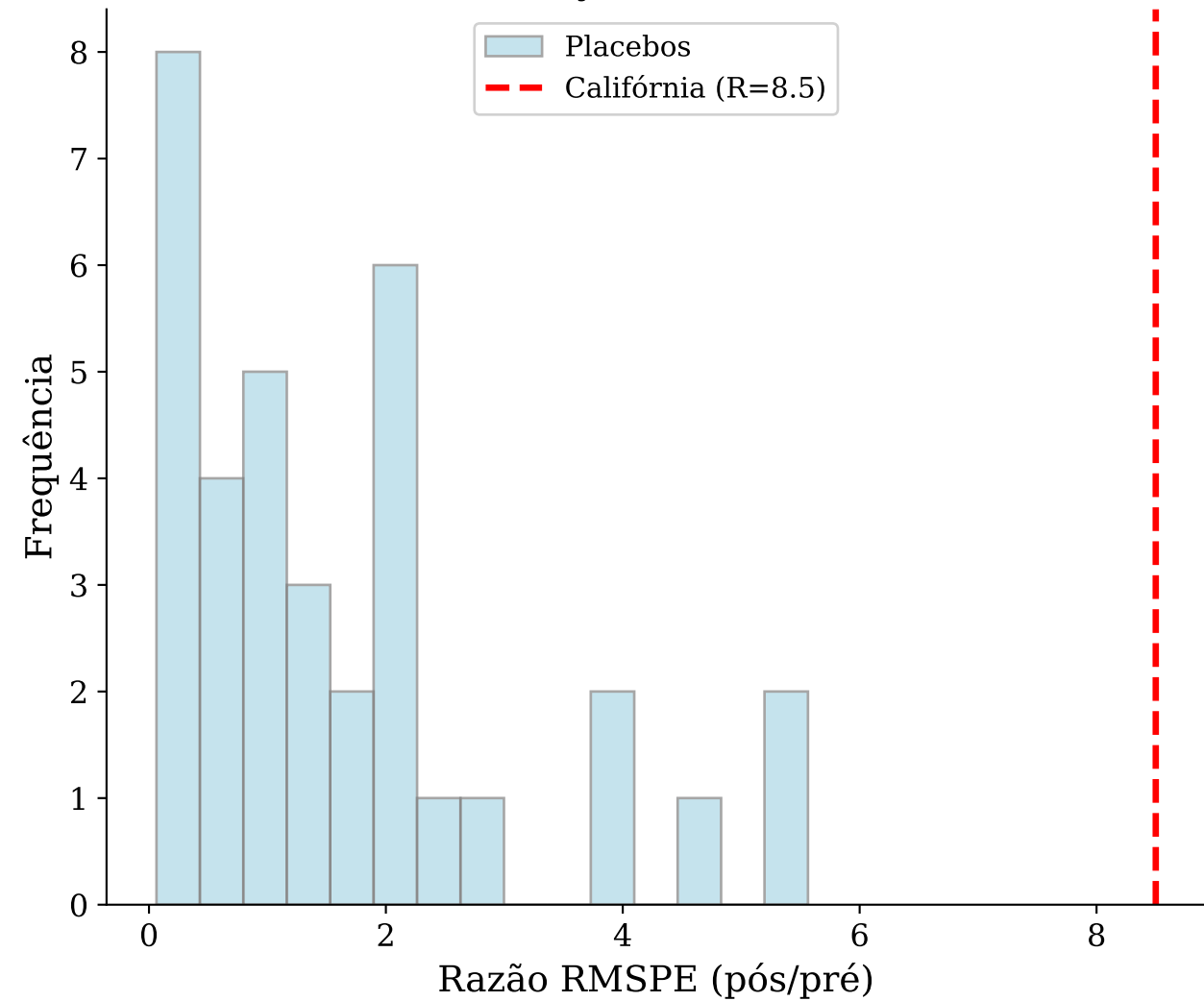
(b) Distribuição da razão RMSPE
