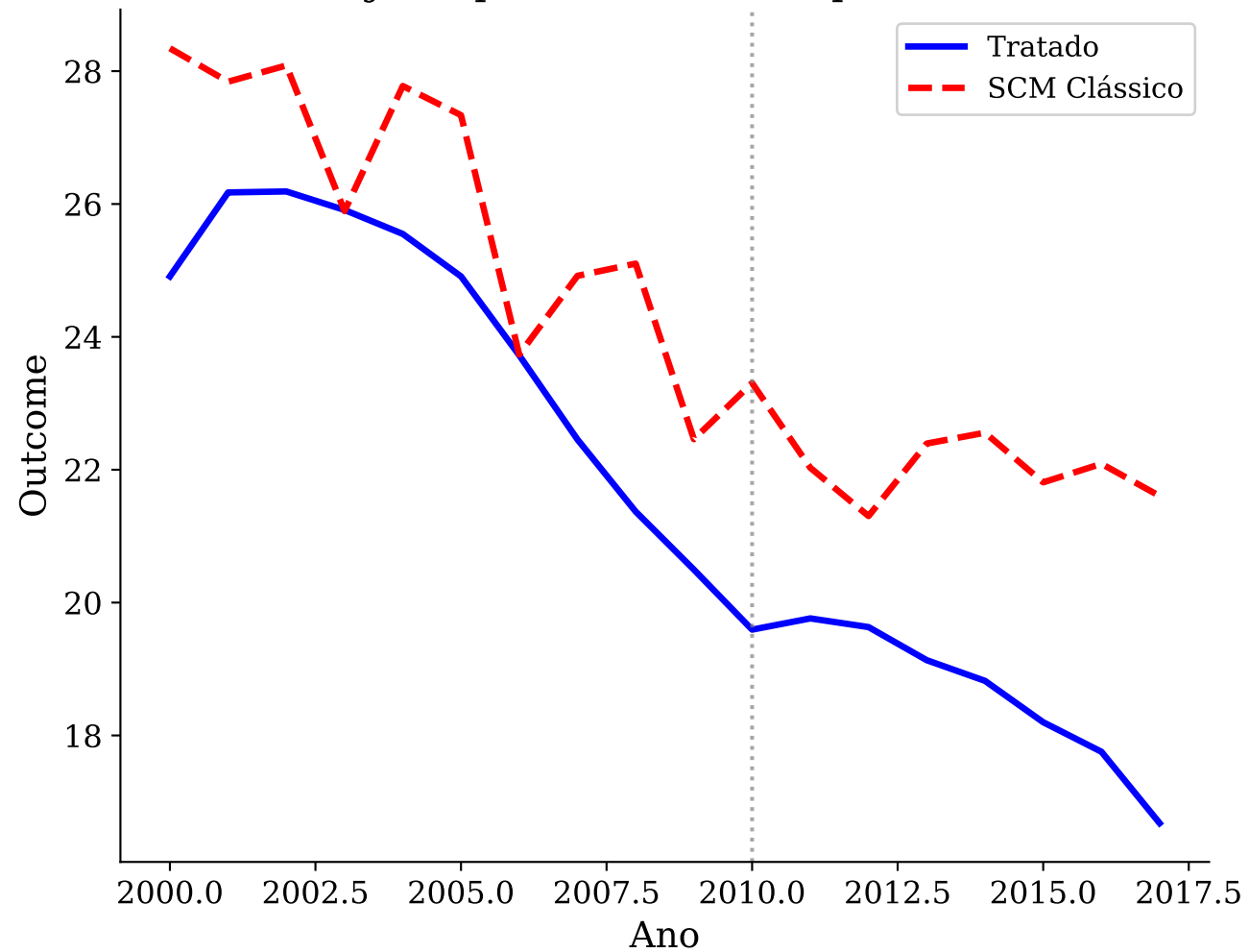
(a) SCM Clássico: ajuste pré-tratamento imperfeito
