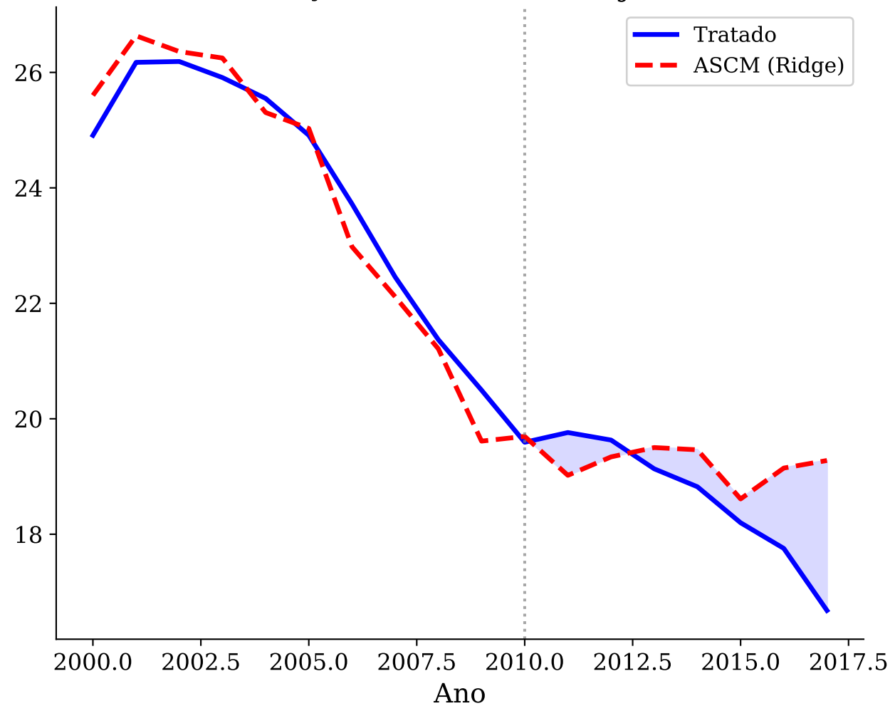
(b) ASCM (Ridge): correção de viés melhora ajuste
