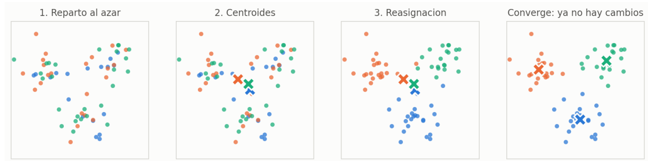
Figura 8: Los cuatro pasos, con tres grupos
