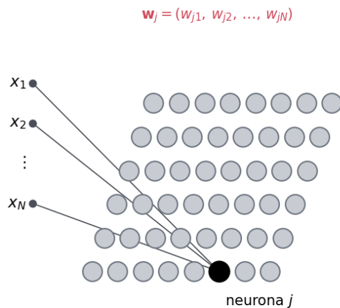
Figura 1: Reconstrucción de las diapositivas 4 a 8. Izquierda: el plano de neuronas y las conexiones. Derecha: la competencia.
