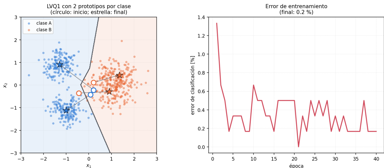
Figura 13: Corrida real: 600 patrones, 4 prototipos, 40 épocas.
