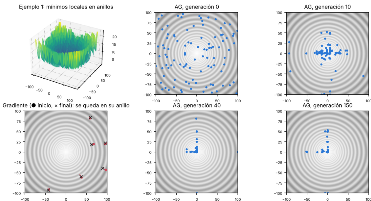
Figura 13: Una superficie con mínimos locales en anillos concéntricos y el mínimo global en el centro. Abajo a la izquierda: seis descensos por gradiente, cada uno queda en su anillo. A la derecha: la población del algoritmo genético en las generaciones 0, 10, 40 y 150. En el pizarrón alcanza con los anillos vistos desde arriba, una flecha de gradiente que queda en un anillo y una nube de puntos que se va juntando en el centro.
