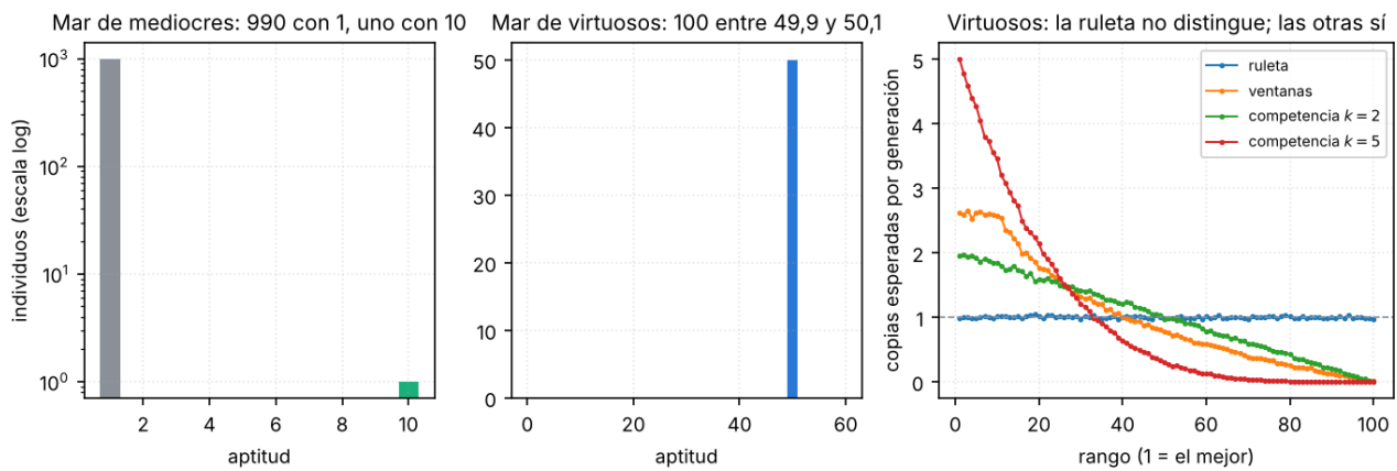
Figura 8: Izquierda y centro: los histogramas de los dos mares. Derecha: copias que espera cada individuo en el mar de virtuosos según el método de selección. La ruleta le da al mejor 0,98 copias, lo mismo que al peor; los otros métodos sí lo distinguen.
