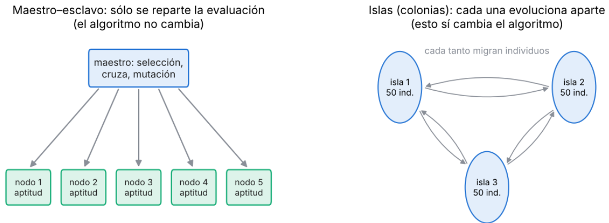
Figura 15: Maestro-esclavo e islas.
