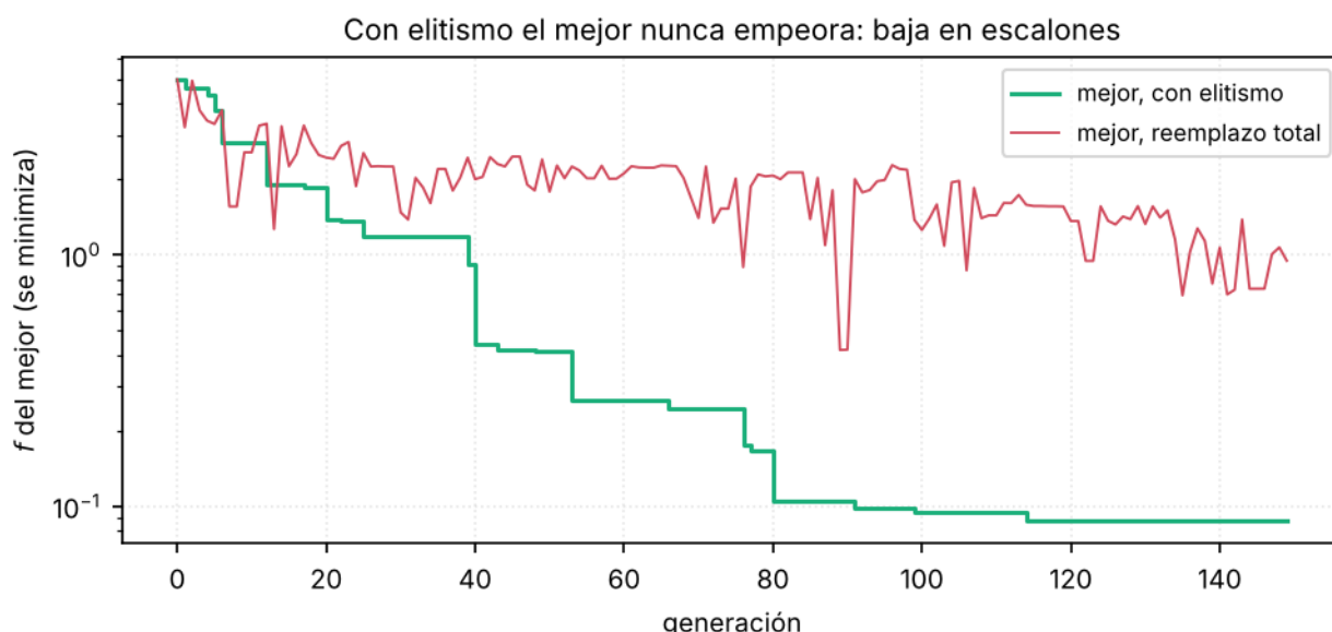
Figura 12: El mismo algoritmo con y sin elitismo. Con elitismo el mejor empeoró 0 veces en 20 corridas de 150 generaciones; sin elitismo, una mediana de 64 veces por corrida. En el pizarrón: una escalera que sólo baja (o sube, si se maximiza) contra una curva que oscila.
