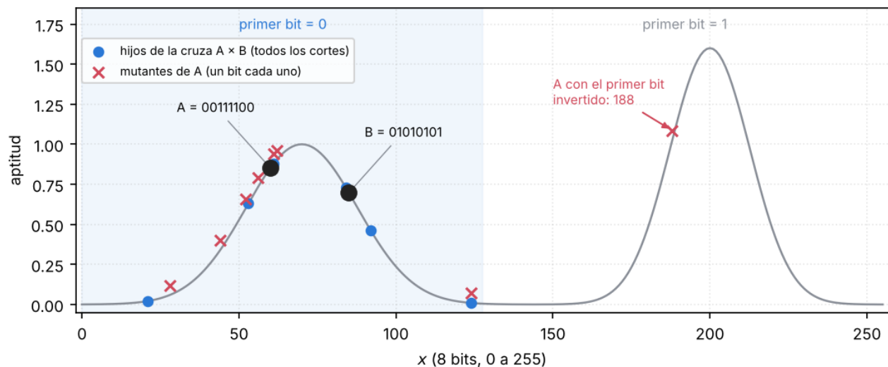
Figura 11: Una variable de 8 bits y una aptitud con dos lomas. Los padres A y B están en la loma de la izquierda y los dos empiezan con 0. Todos sus hijos posibles (puntos azules) quedan en esa loma. Los mutantes de A (cruces) quedan cerca, salvo el del primer bit, que salta a 188, en la otra loma. Es el dibujo para explicar exploración y explotación.
