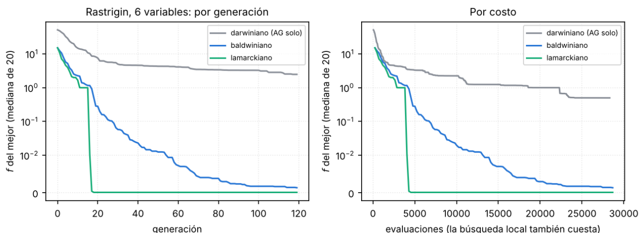
Figura 17: Función de Rastrigin con 6 variables (muchos mínimos locales). La búsqueda local son 3 pasos de gradiente por individuo y por generación, y se cuentan en el costo.
