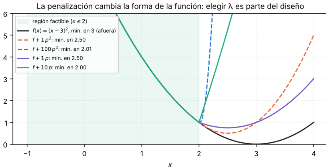
Figura 16: Minimizar (x-3)^2 con la restricción x \leq 2 . El mínimo verdadero, respetando la restricción, es x = 2 . Con penalización cuadrática, aun con \lambda = 100 , el mínimo de la función penalizada queda en 2,01, fuera de lo permitido. Con penalización lineal y \lambda = 10 cae justo en 2.
