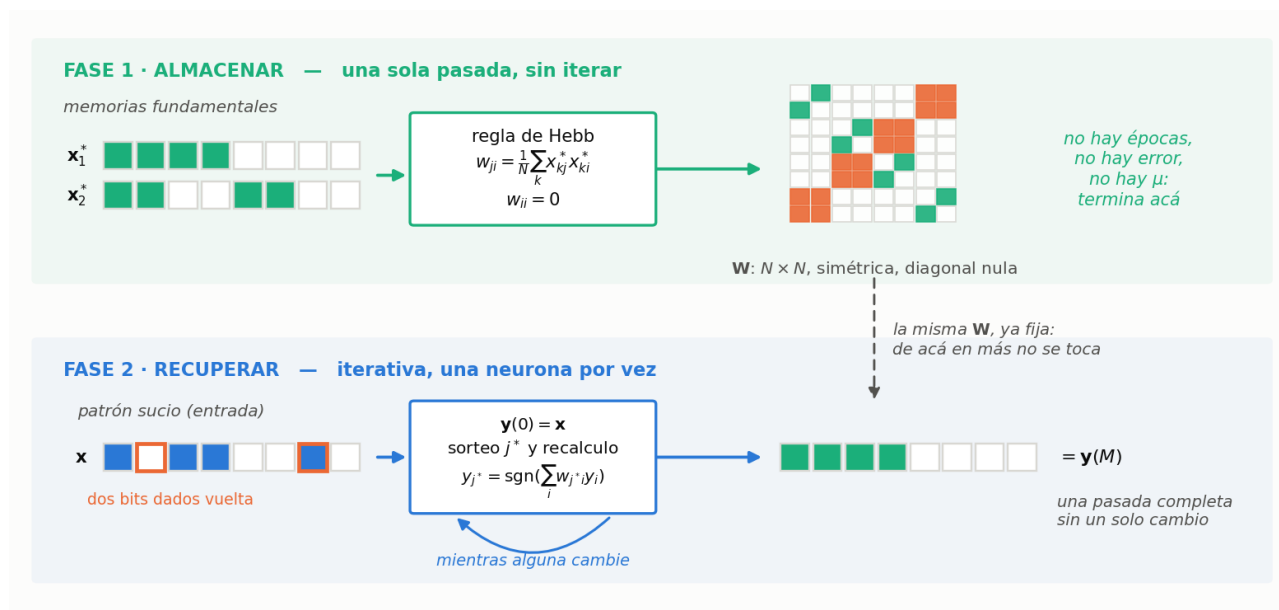
Figura 4: Escribir la memoria es una cuenta; leerla es dejar correr la red. Los dos carriles no se mezclan: cuando empieza el de abajo, \mathbf{W} ya está fija.
