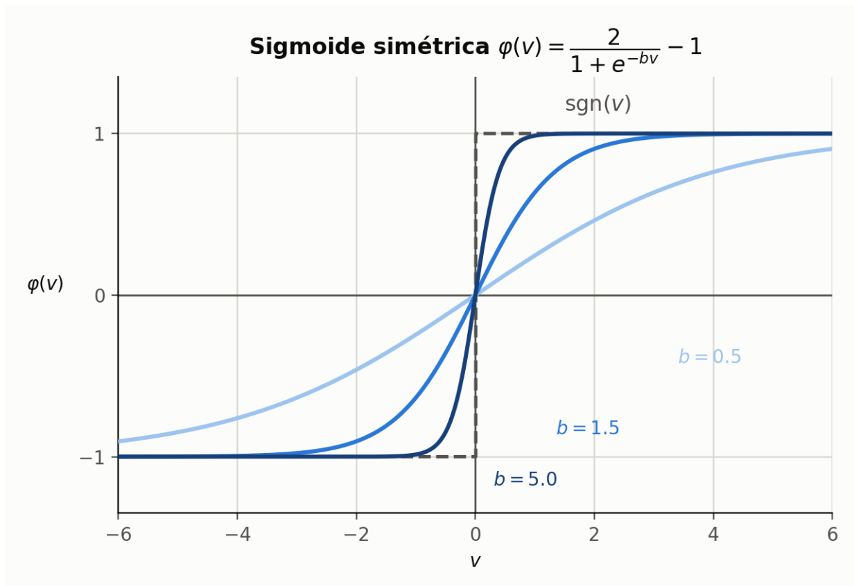
Figura 3: La sigmoide simétrica para tres valores de b , con \text{sgn} punteada como referencia.
