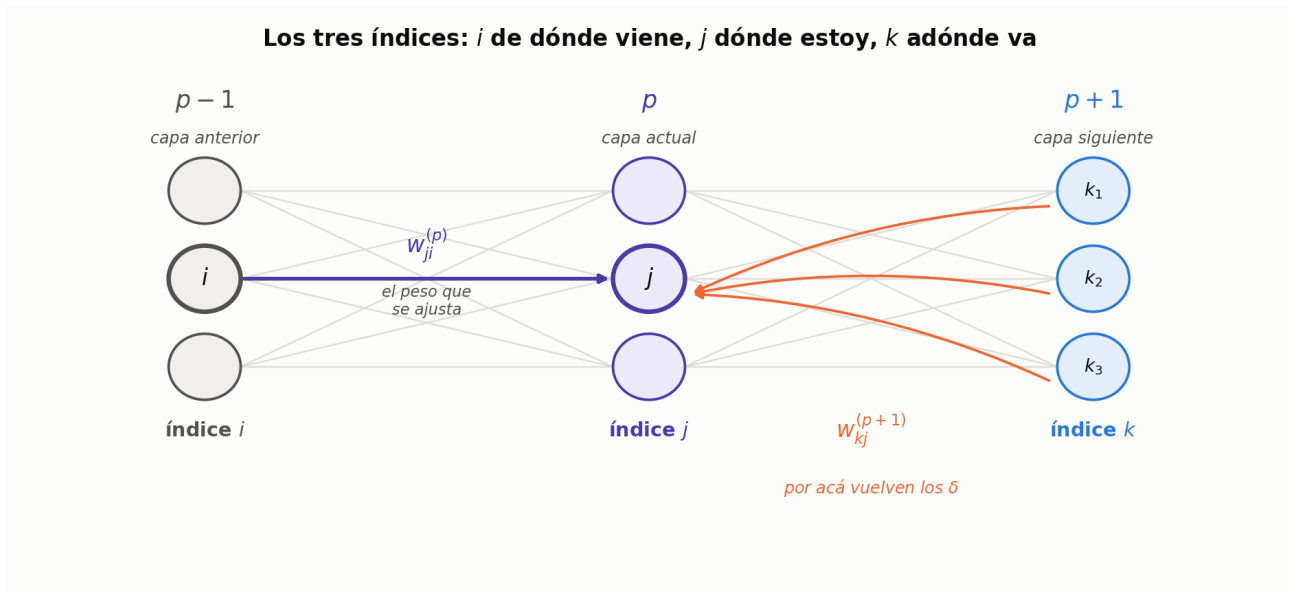
Figura 7: Cada índice vive en una capa distinta. Confundirlos es el error más común de toda la unidad.
