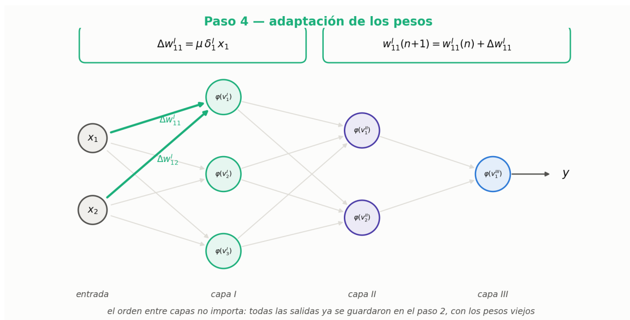
Figura 14: Recién acá cambian los pesos, y todos con los mismos valores guardados del paso 2.
