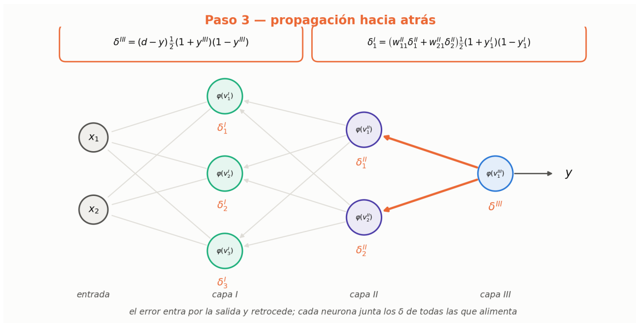
Figura 13: El error entra por la salida y retrocede convertido en \delta .
