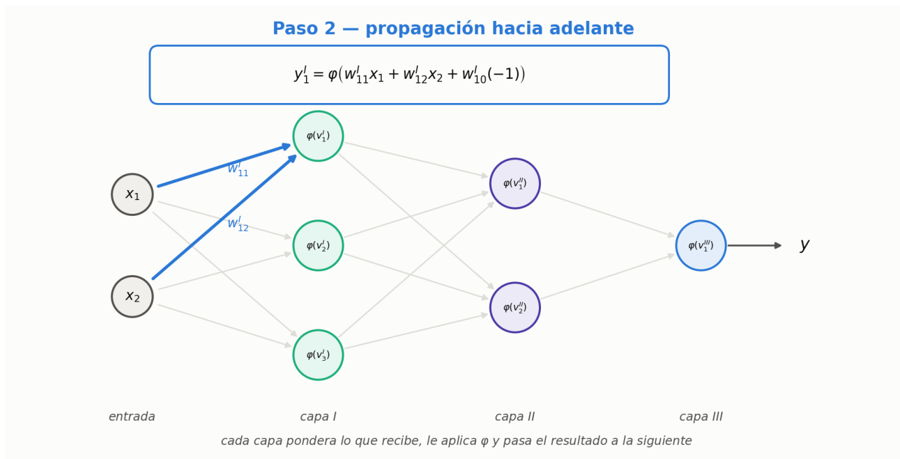
Figura 12: Se entra un patrón y se calcula la salida de cada neurona, capa por capa.
