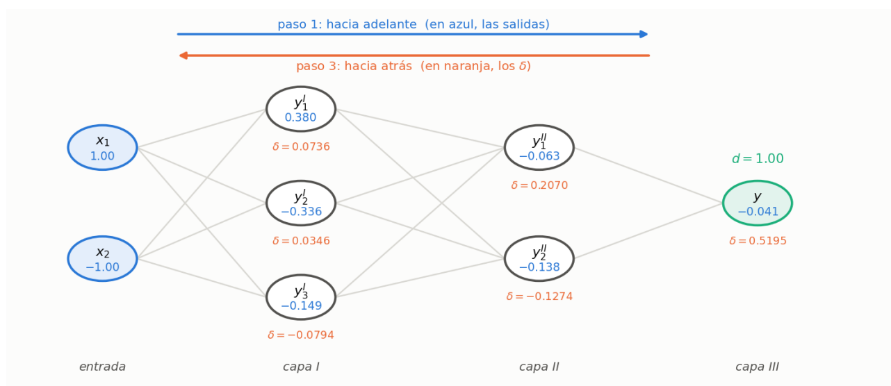
Figura 15: La red del ejemplo: en azul los valores del paso 1, en naranja los \delta del paso 3
