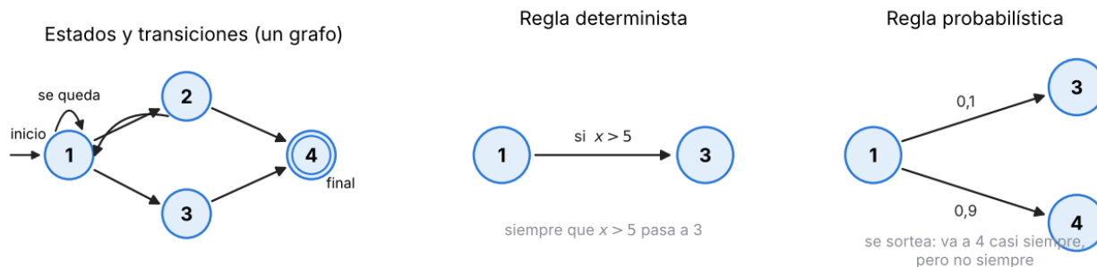
Figura 2: Izquierda: un autómata de cuatro estados, con estado inicial y final (1 es el inicial, 4 el final). Centro y derecha: los dos tipos de regla de transición.
