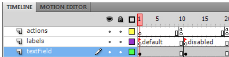
그림 13: Label 타임라인.
