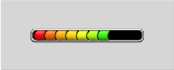
59: StatusIndicator
