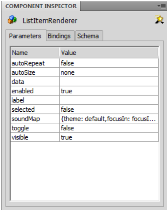
ListItemRenderer
