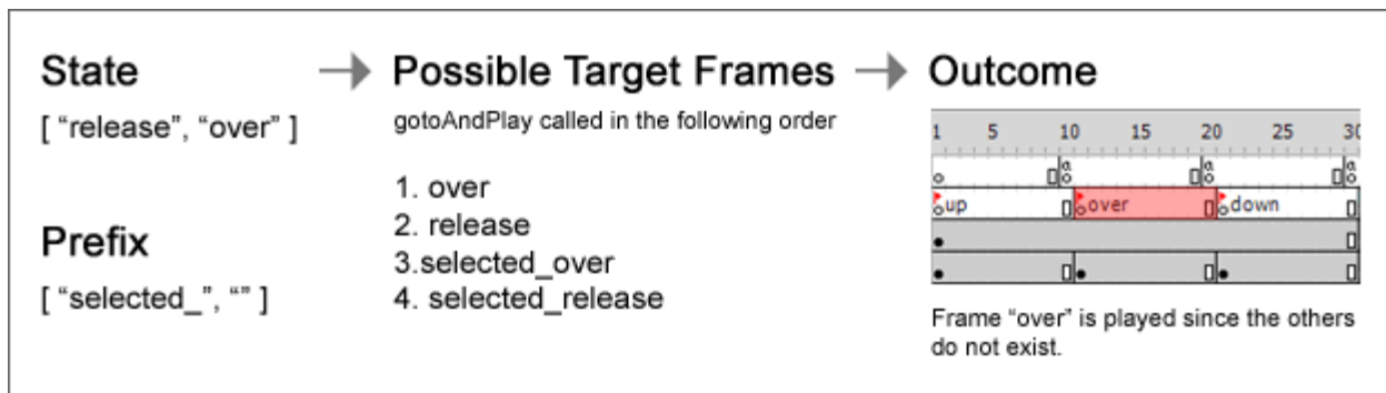
그림 61: 올바른 재생 키프레임을 결정하는데 사용되는 프로세스
