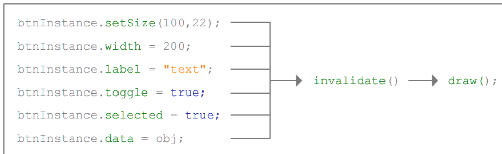
그림 63: CLIK 컴포넌트는 특정 속성이 변경되면 자동적으로 무효화한다.
