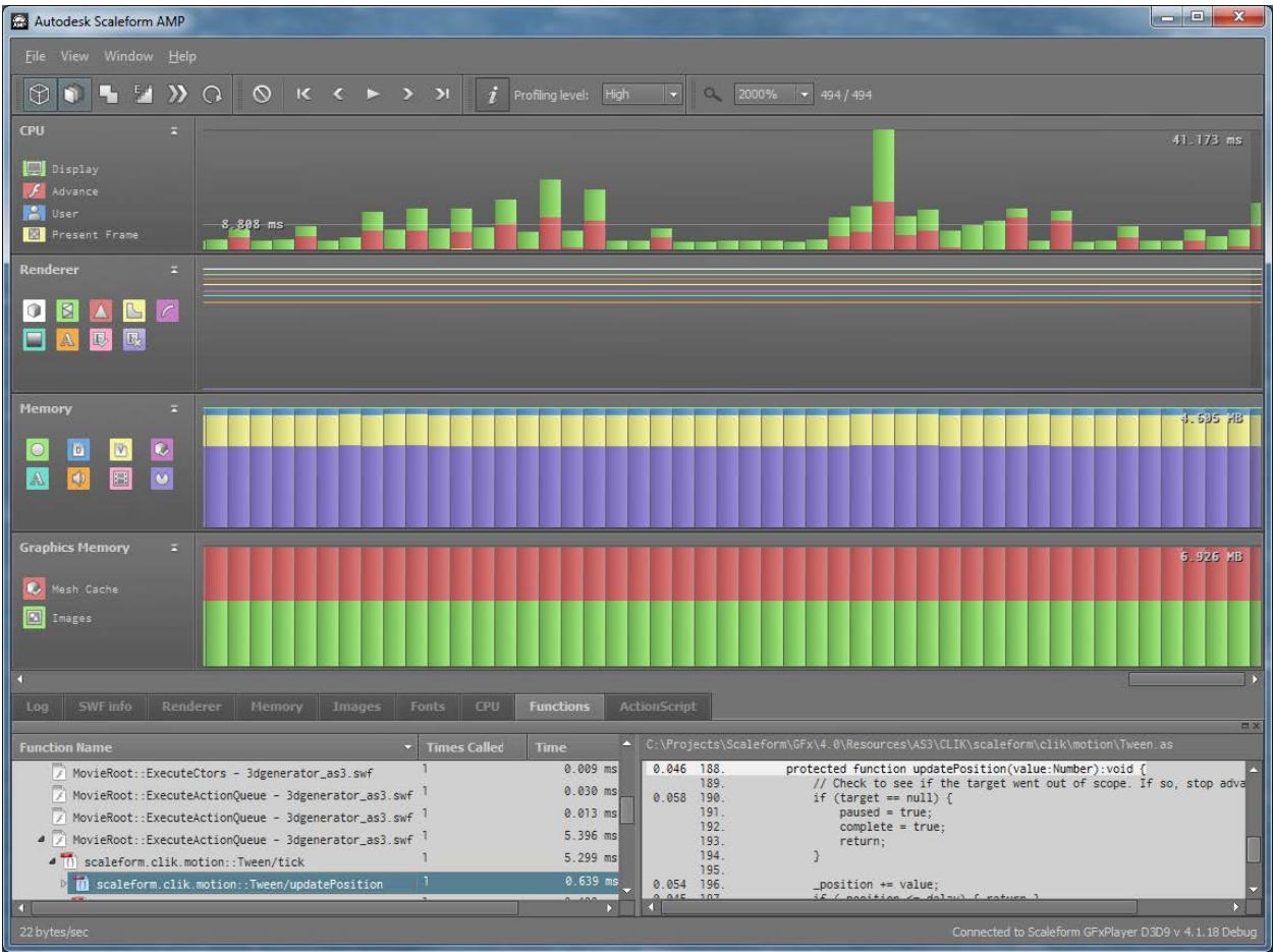
그림 1: Scaleform AMP
