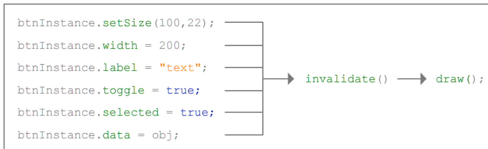
그림 60: CLIK 컴포넌트는 특정 속성이 변경되면 자동적으로 무효화한다.
