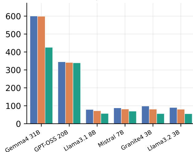
Output tokens
