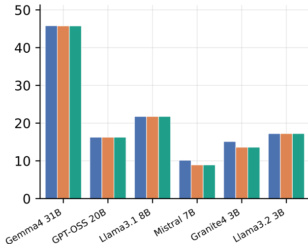
VRAM (GB)
