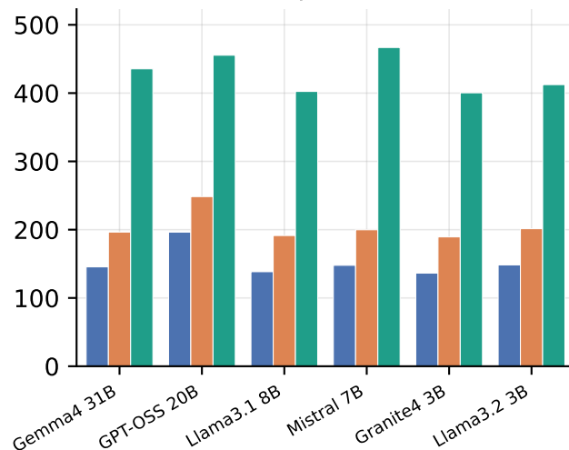
Prompt tokens
