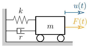
Abbildung 1: Einmasseschwinger
