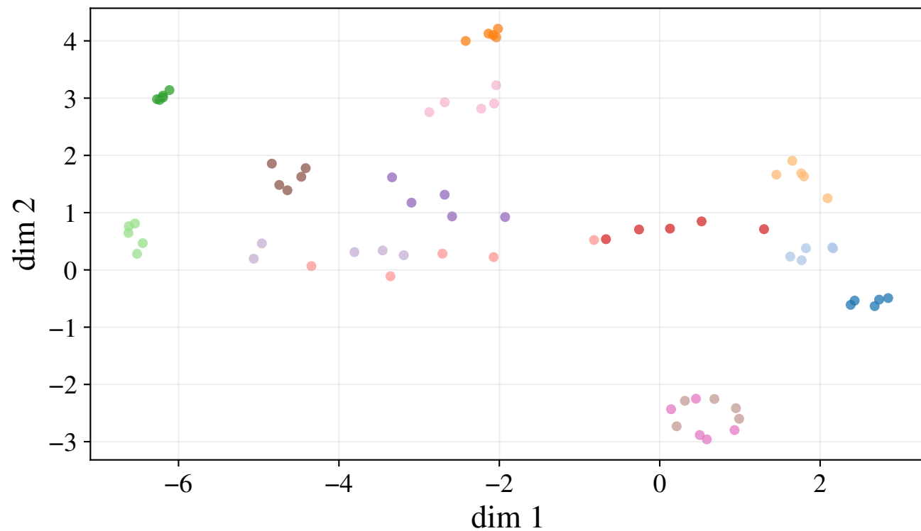
t-SNE
