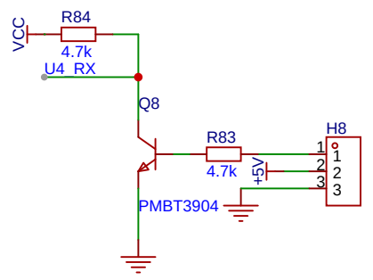
大疆DBUS接口
