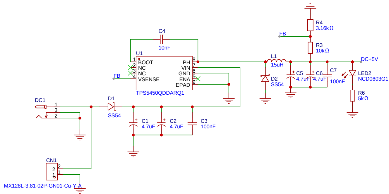
DCDC电路
