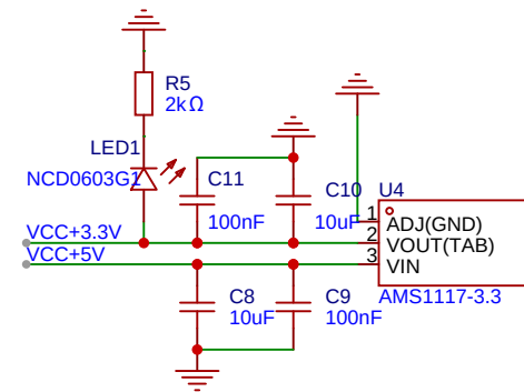
LDO电路
