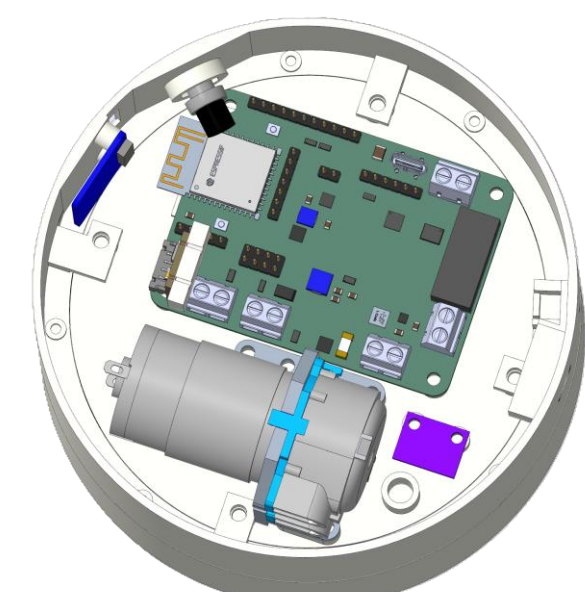
Abb. 3: Querschnitt mit Blick in die Elektronikammer
