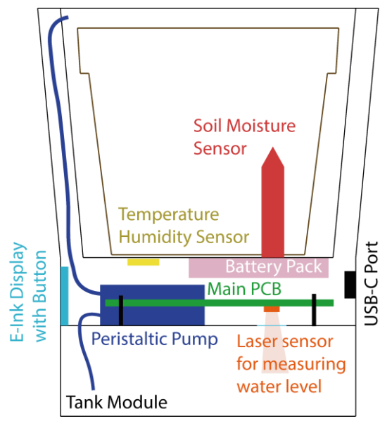
Abb. 5: Schematische Skizze
