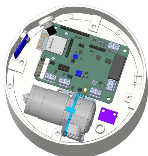
Abb. 6: Querschnitt mit Blick in die Elektronikammer
