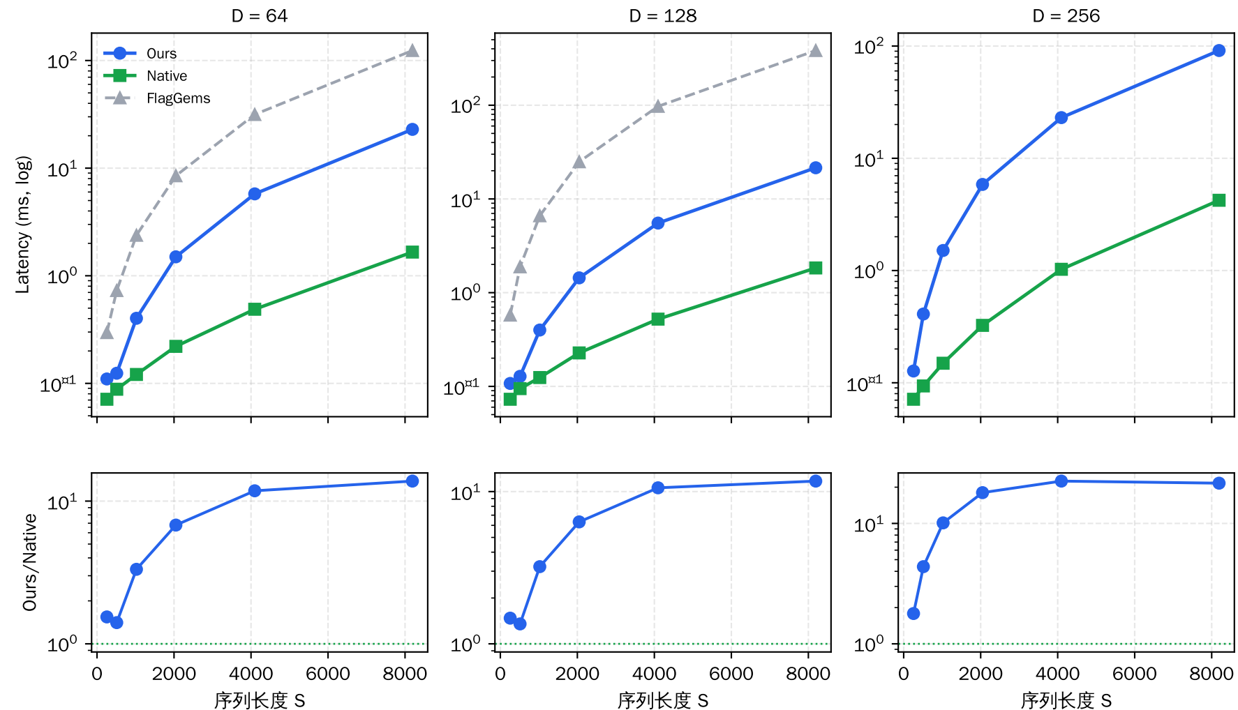
多尺度性能扫描: 延迟随 S 变化 (fp16, causal, H=16) 上:绝对延迟 下:与原生比值
